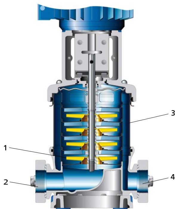
Рис. 3: Сечение
