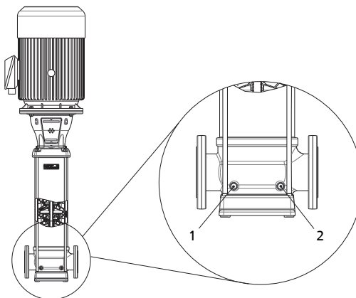
Рис. 11: Соединения для выполнения опорожнения насоса
