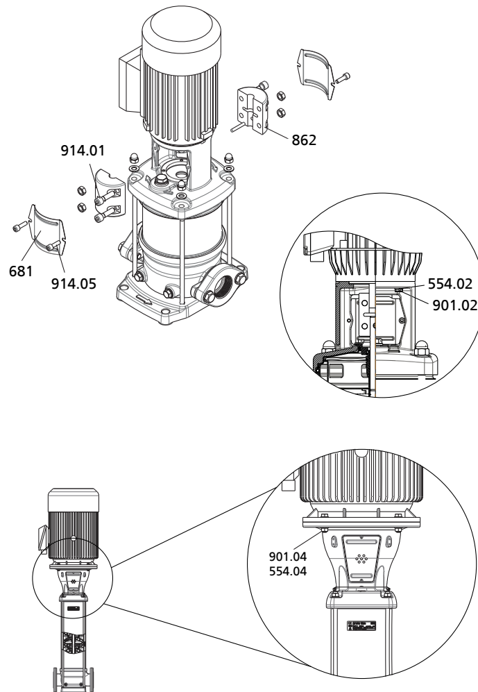
Рис. 12: Демонтаж двигателя
