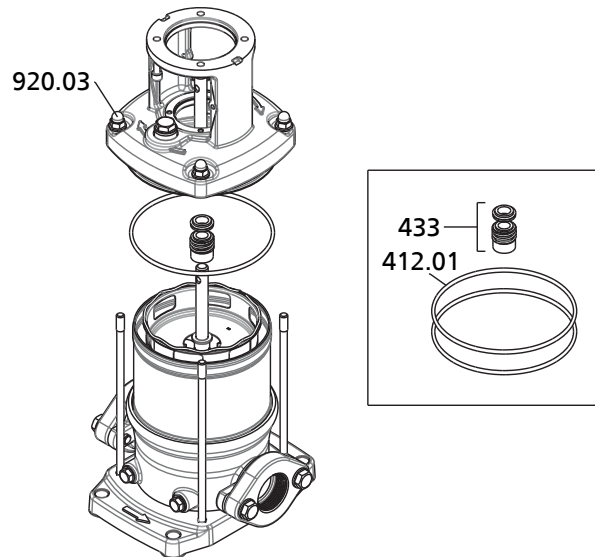
Рис. 13: Демонтаж торцевого уплотнения
