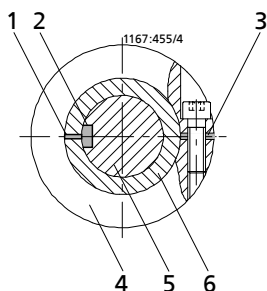
Рисунок 9: Установка конца вала двигателя на вал
