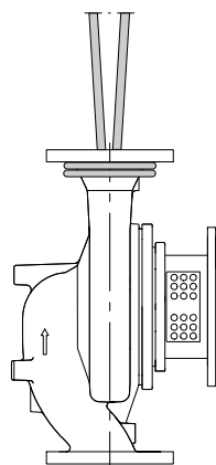
Рисунок 2: Транспортировка насоса
