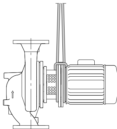
Рисунок 1: Транспортировка насосного агрегата
