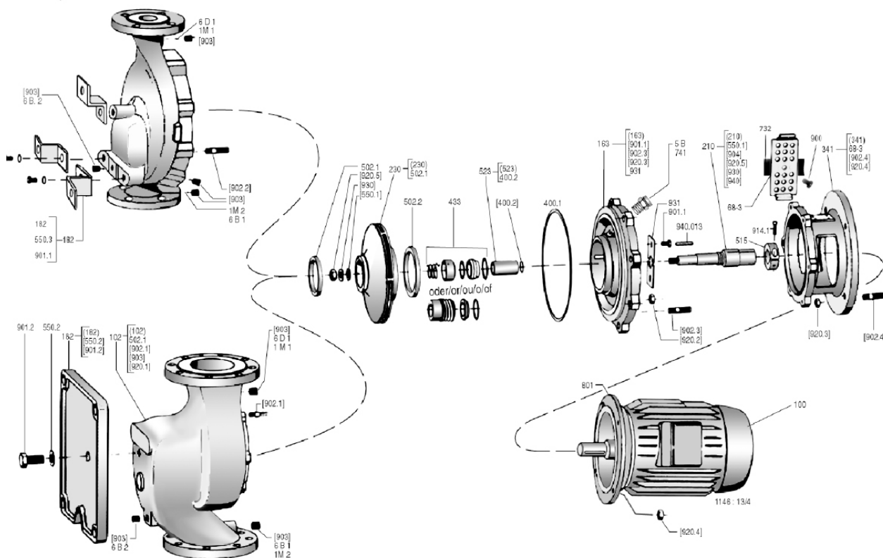
Рисунок 12: Стандартное торцевое уплотнение и резьбовая напорная крышка
