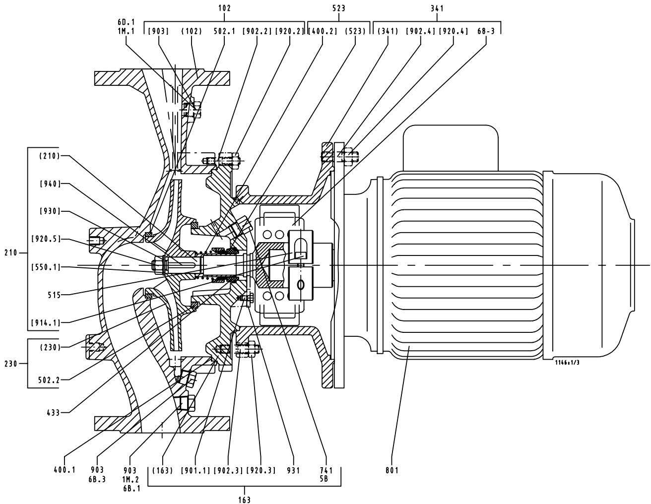
Рисунок 14: Стандартное торцевое уплотнение и резьбовая напорная крышка
