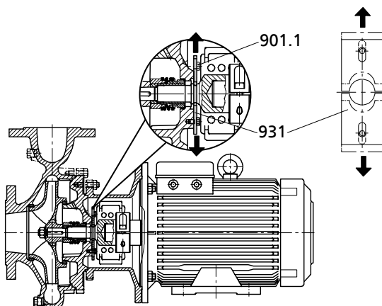
Рисунок 10: Удаление стопорных пластин
