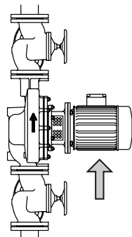
Рисунок 5: Обеспечить опирание двигателя
