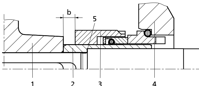
Рисунок 8: Установочный размер b торцевого уплотнения
