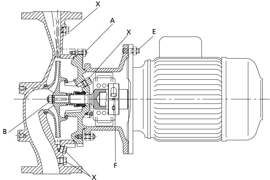
Рисунок 11: Места затяжки винтов
