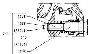
Рисунок 15: Крепление рабочего колеса при WE 35
