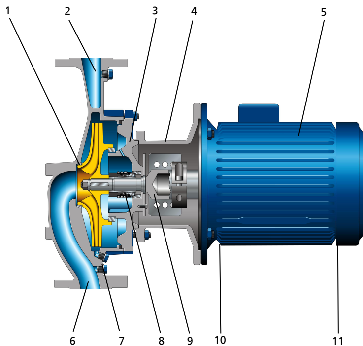
Рисунок 4: Сечение
