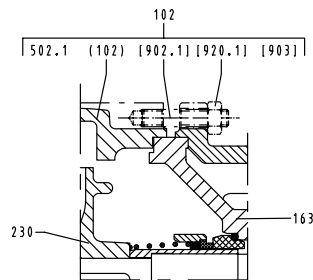
Рисунок 16: Крепление напорной крышки
