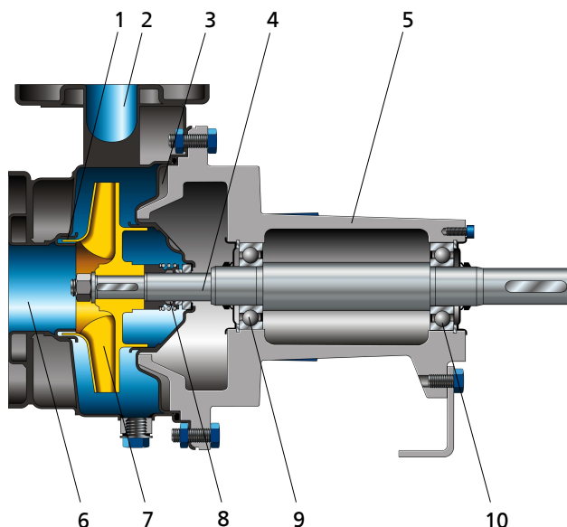
Рисунок 5: Вид в разрезе
