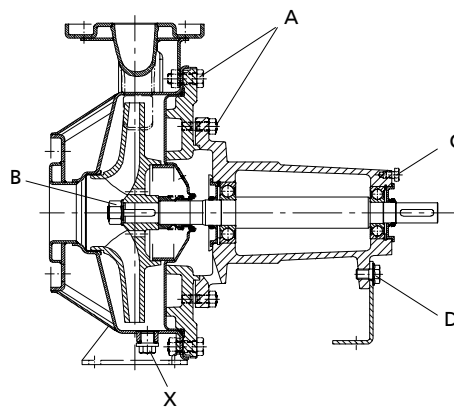
Рисунок 17: Позиции затяжки винтов диаметр рабочего колеса 250, 50-200, 65-200, 80-200
