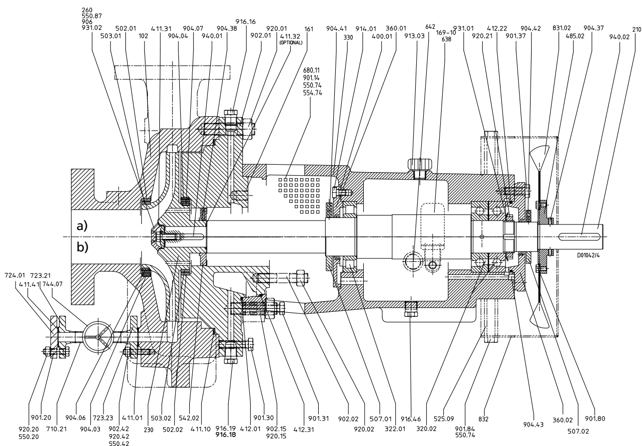
Рис. 16: Корпус подшипников V06 и V07, а) без охлаждения и б) с охлаждением
