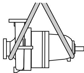
Рис. 2: Транспортировка насоса
