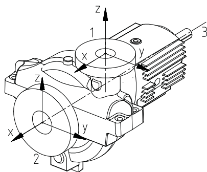
Рис. 8: Система координат действующих сил или моментов
