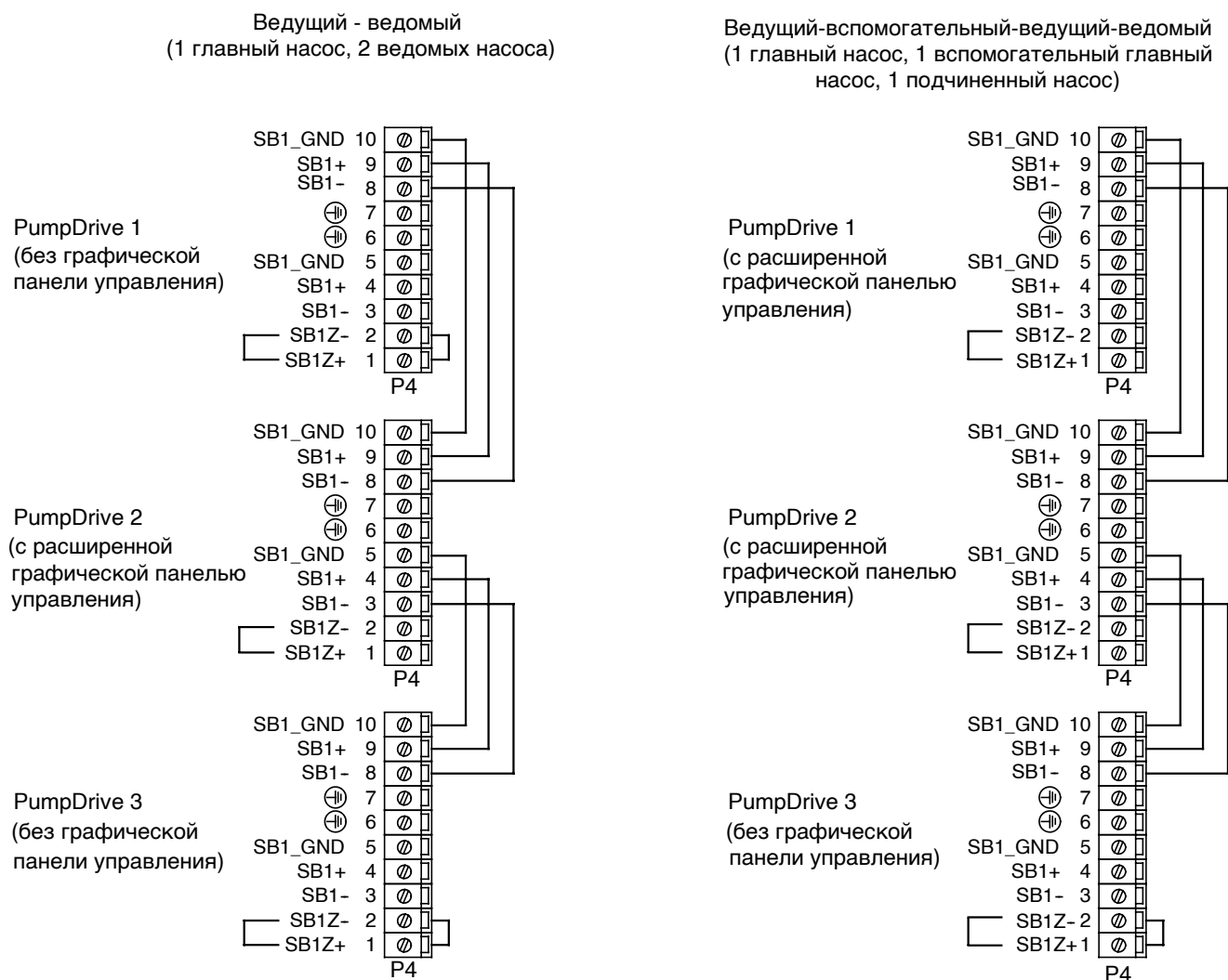
Рис. 16: Монтажная схема локальной шины KSB "Local-Bus" в режиме ведущий-ведомый и ведущий-вспомогательный-ведущий-ведомый
