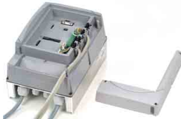
Рис. 14: Снятие крышки клемм управления
