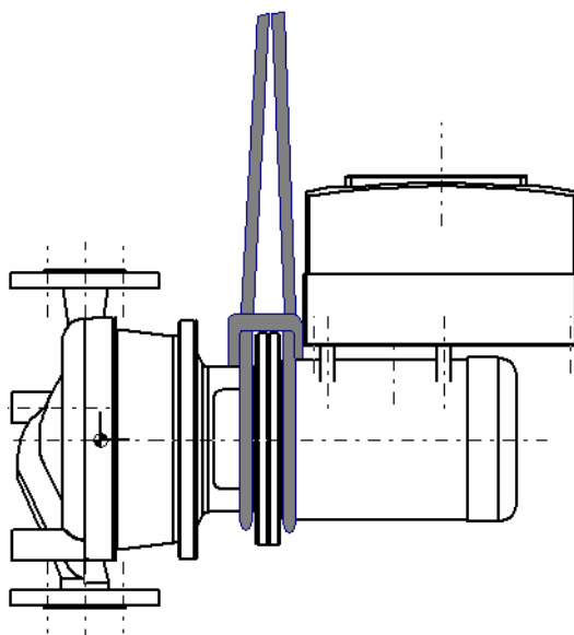
Рис. 2: Транспортировка Etaline/Etabloc PumpDrive
