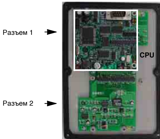
Рис. 21: Стандартное исполнение панели управления
