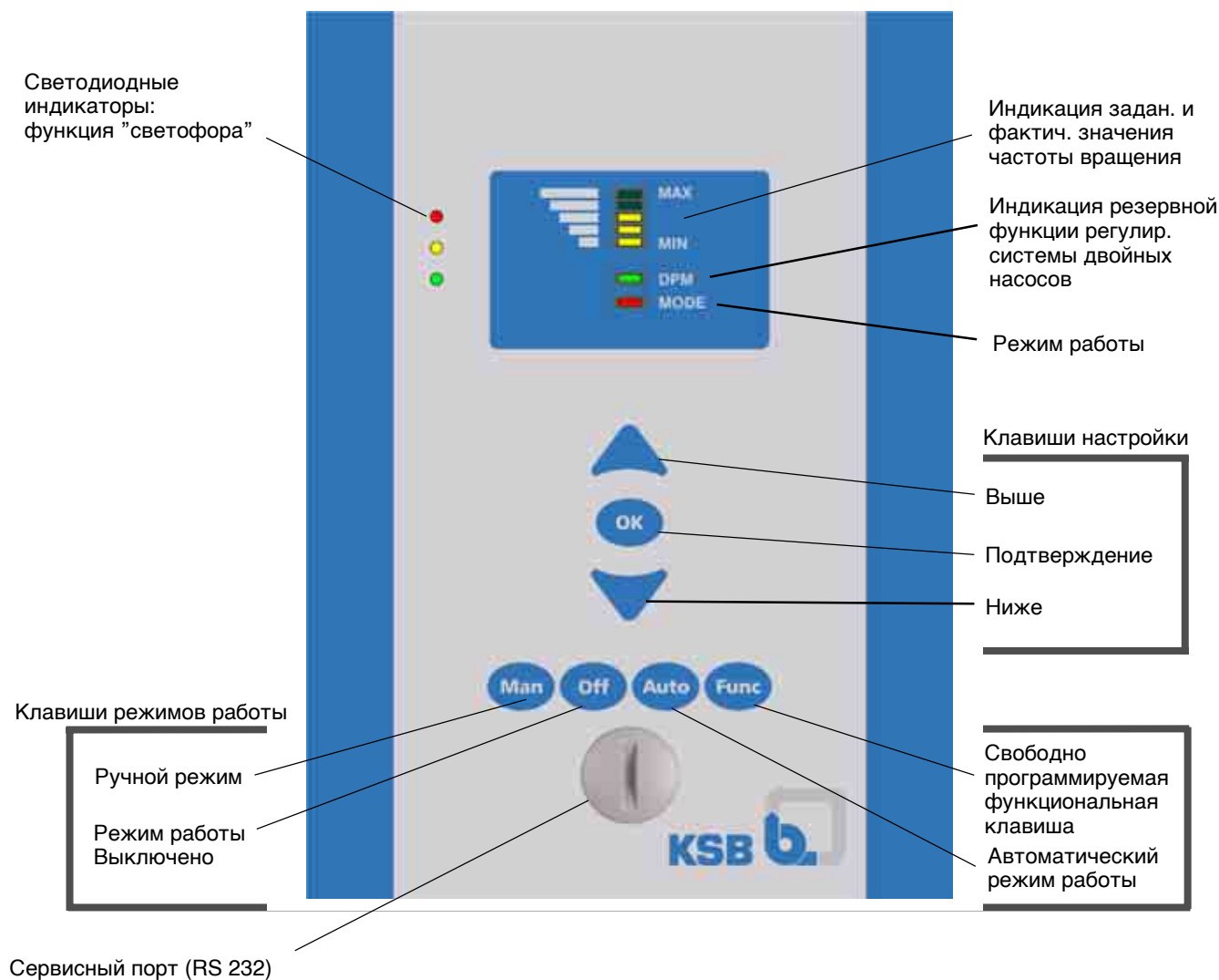
Рис. 7: Стандартная панель управления
