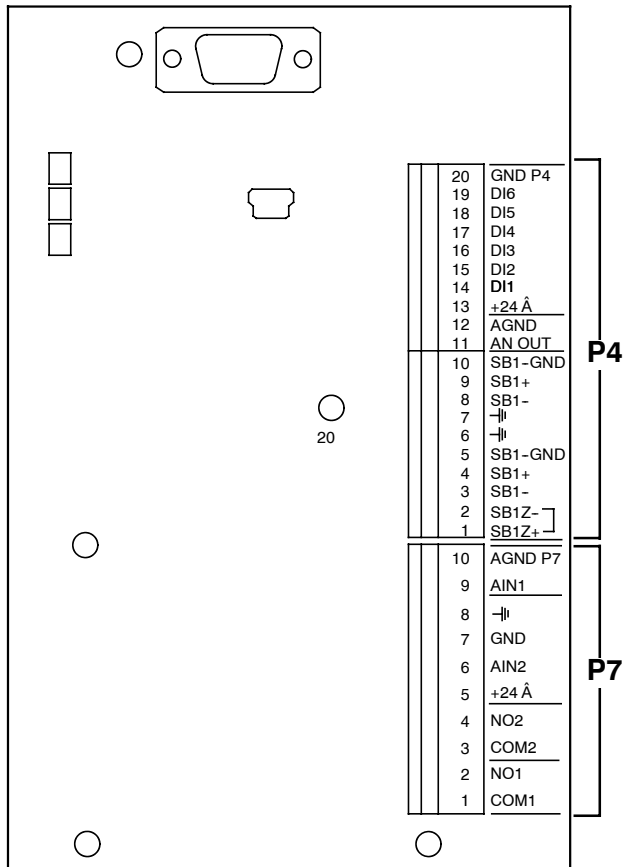
Рис. 15: Входы / выходы клемм управления
