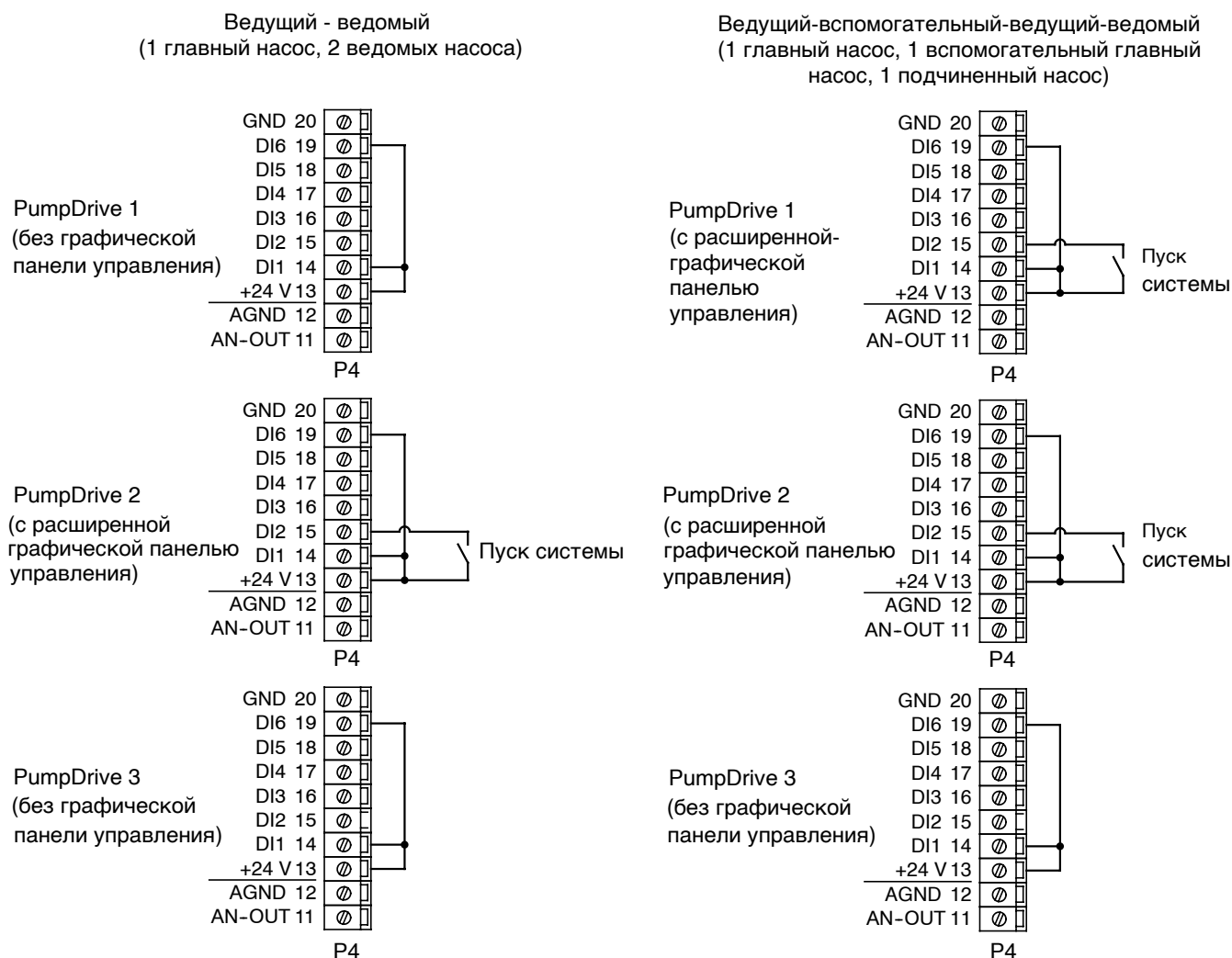
Рис. 17: Электрическая схема для режима ведущий-ведомый и для режима ведомый-вспомогательный-ведущий-ведомый
