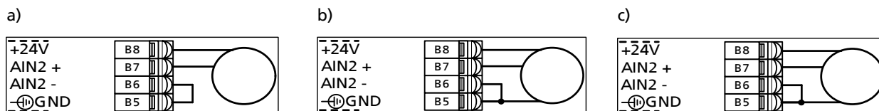
Рис. 52: Подключение чувствительных элементов к дифференциальному аналоговому входу
