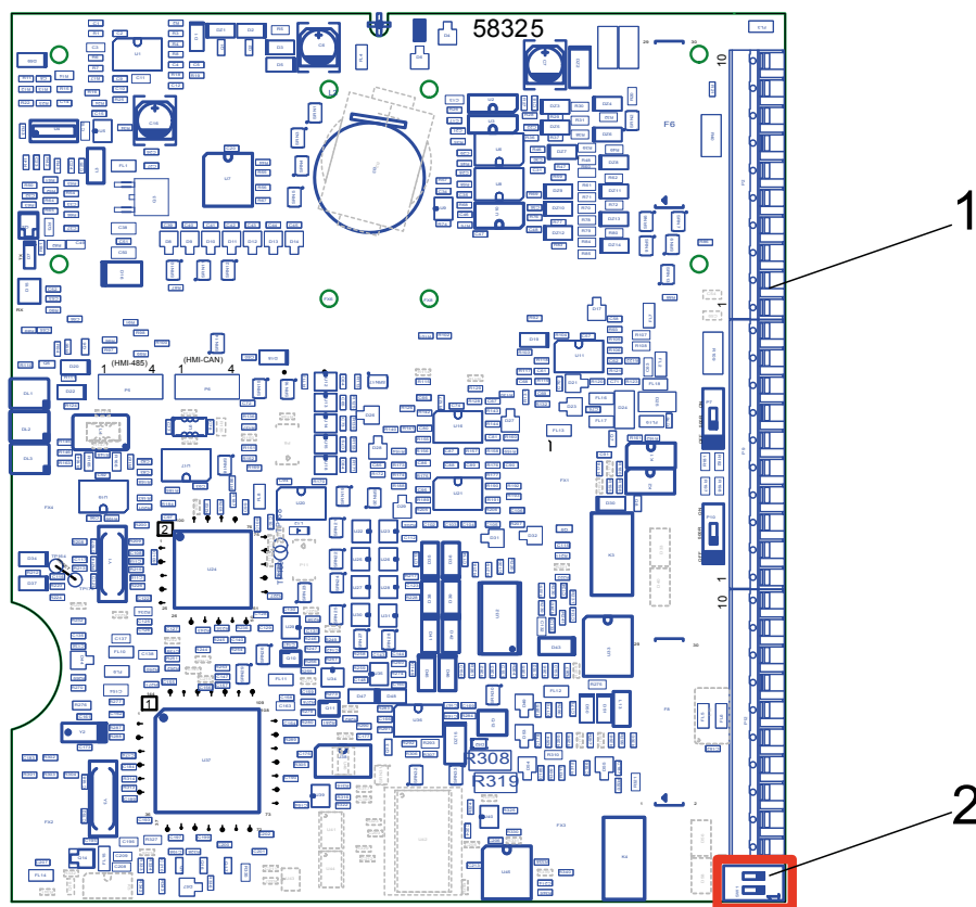
Рис. 88: Положение DIP-переключателя на плате управления
