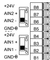
Рис. 86: DIP-переключатель аналоговых входов (заводская настройка)
