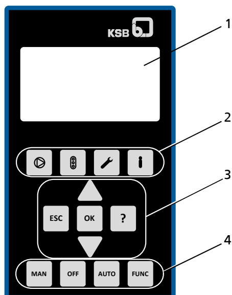
Рис. 54: Графическая панель управления
