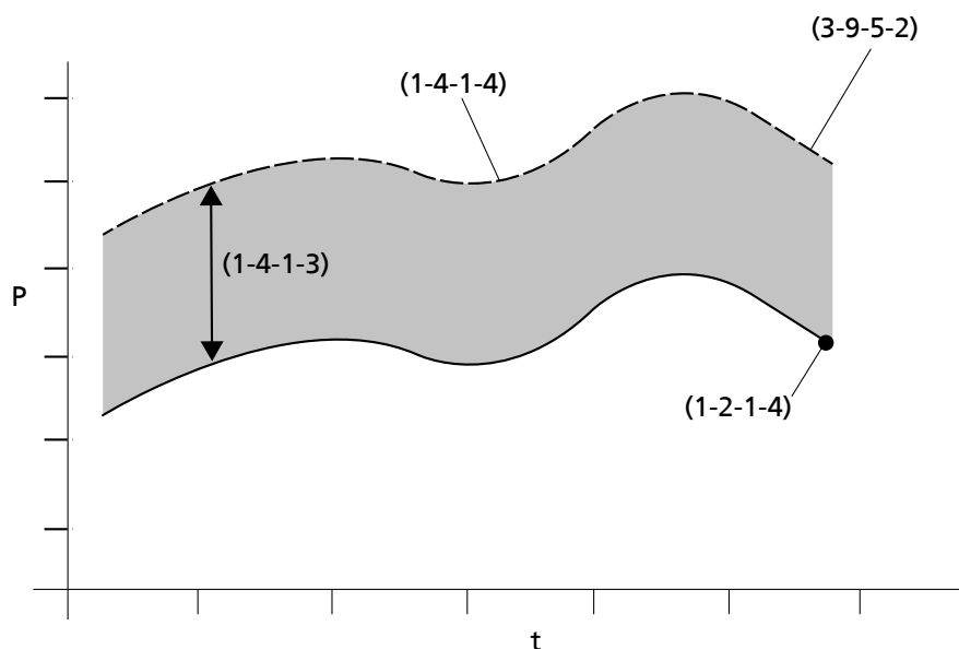
Рис. 80: Экономия электроэнергии с переменной контрольной мощностью
