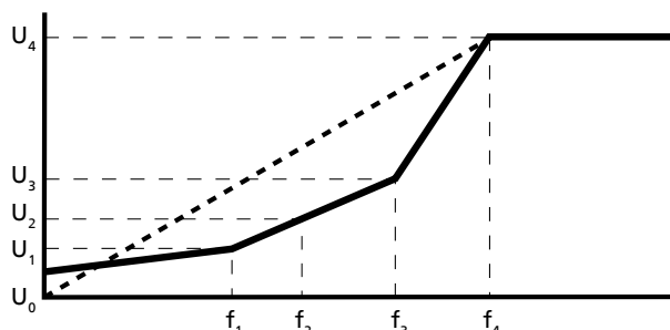
Рис. 60: Вольт-частотная характеристика
