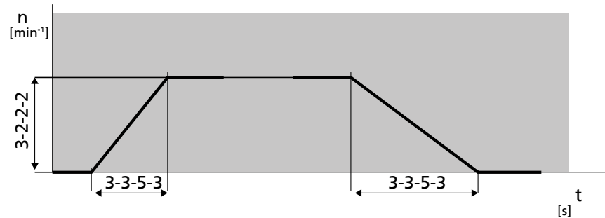
Рис. 82: Линейный сигнал работы
