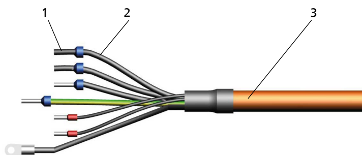
Рис. 9: Устройство кабеля
