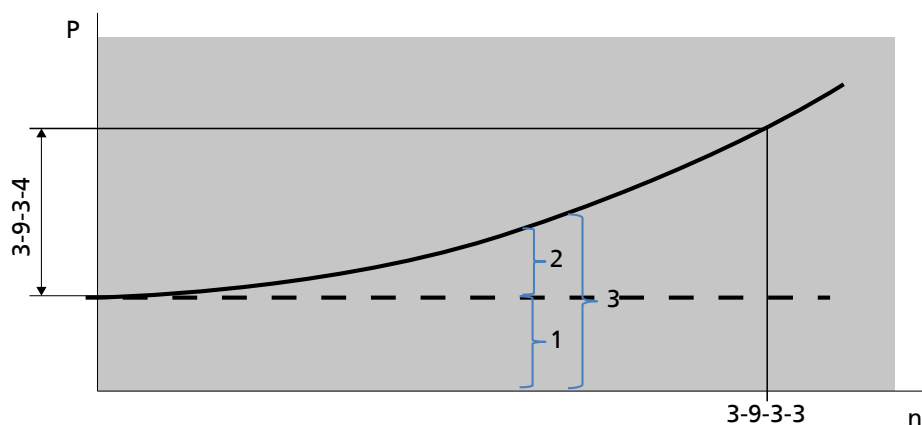
Рис. 75: Форма кривой увеличенного заданного значения при регулировании DFS на основе частоты вращения
