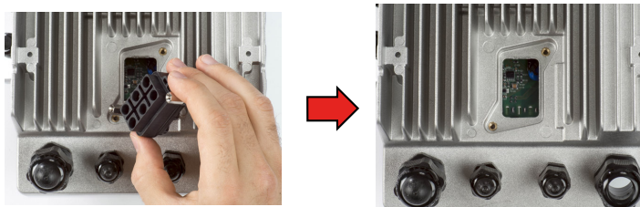
Рис. 23: Снятие разъема двигателя
