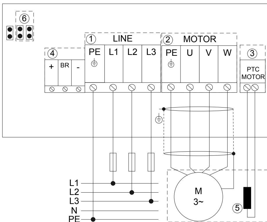
Рис. 19: Подключение к сети питания и двигателю, типоразмер E
