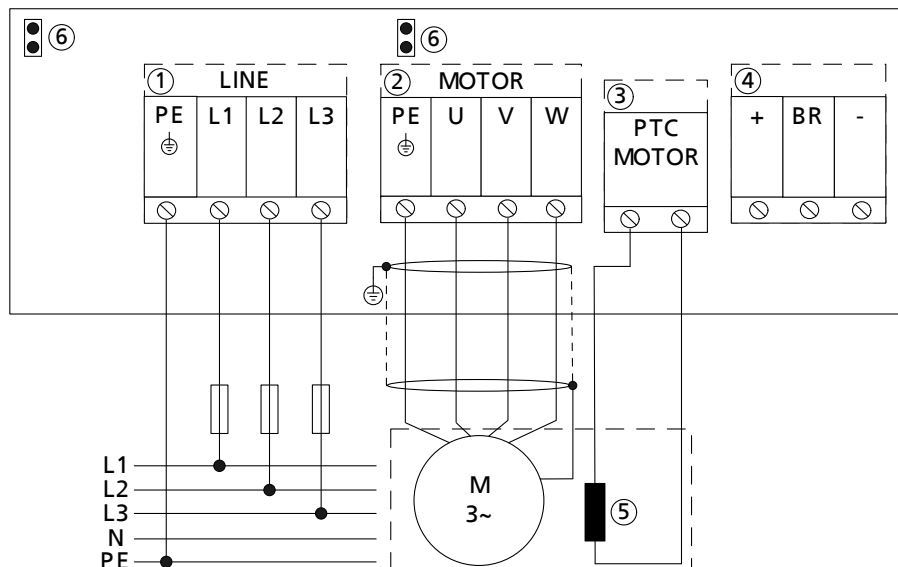
Рис. 16: Подсоединение к сети питания и двигателю, типоразмер В
