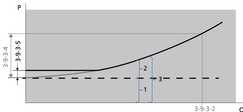
Рис. 74: Кривая изменения повышенного заданного значения при регулировании DFS на основе подачи с минимальным повышением заданного значения (3-9-3-5)
