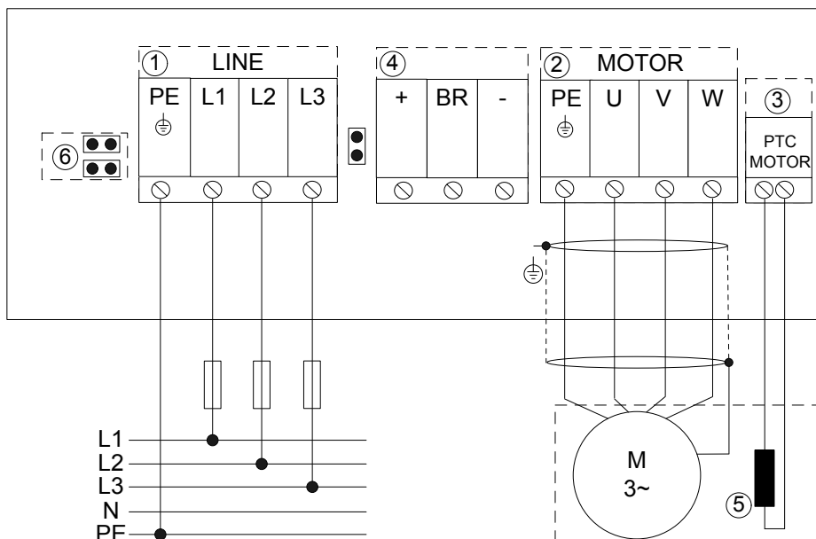
Рис. 18: Подключение к сети питания и двигателю, типоразмер D
