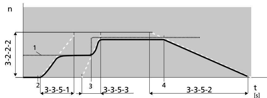
Рис. 83: Пример изменения частоты вращения в режиме ручного регулирования
