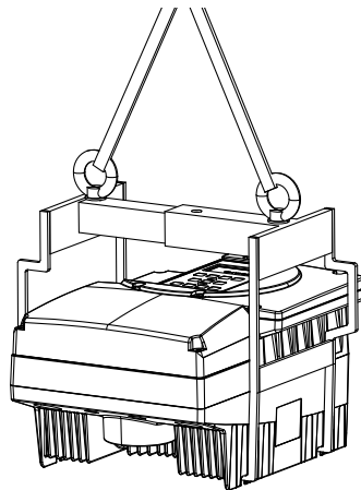
Рис. 5: Транспортировка частотного преобразователя с помощью подъемного устройства
