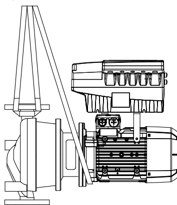
Рис. 1: Транспортировка моноблочного агрегата
