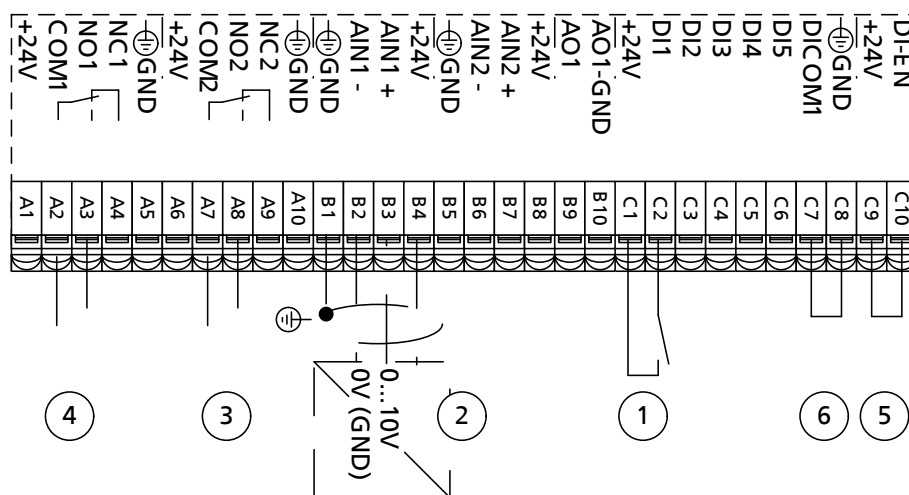
Рис. 61: Схема подключений для режима ручного регулирования (заштрихованный участок = по запросу)
