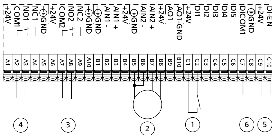
Рис. 63: Схема подключений для режима автоматического регулирования (заштрихованный участок = по запросу)
