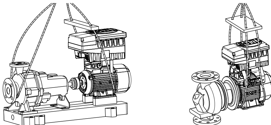
Рис. 2: Транспортировка горизонтального насосного агрегата
