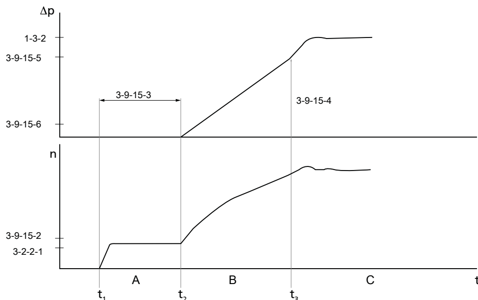
Рис. 85: Функция заполнения трубопровода, временная диаграмма
