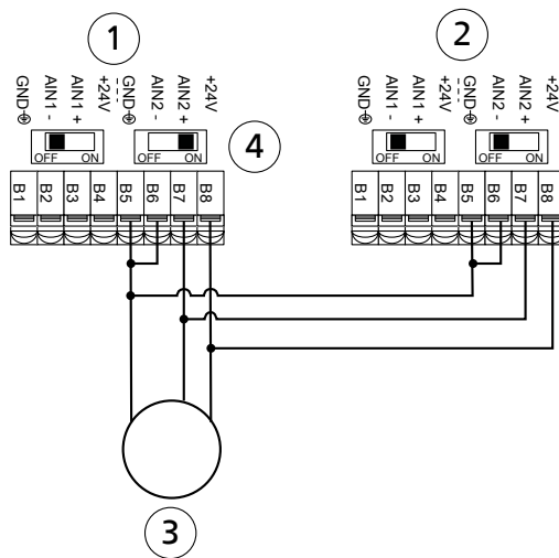
Рис. 87: Пример прохождения сигнала 4-20 мА
