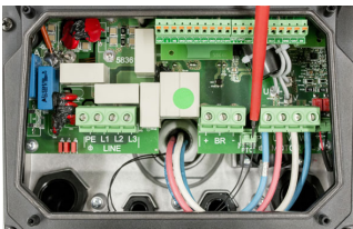
Рис. 29: Подключение кабелей двигателя
