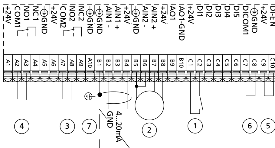
Рис. 64: Схема подключений для режима автоматического регулирования (заштрихованный участок = по запросу)
