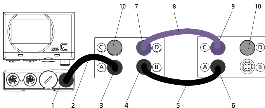
Рис. 38: Подсоединение PumpMeter в двухнасосном/многонасосном режиме
