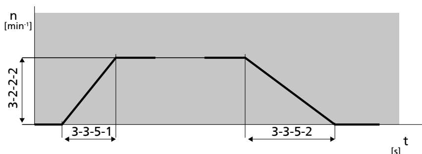
Рис. 81: Линейный сигнал пуска (слева) и линейный сигнал останова (справа)
