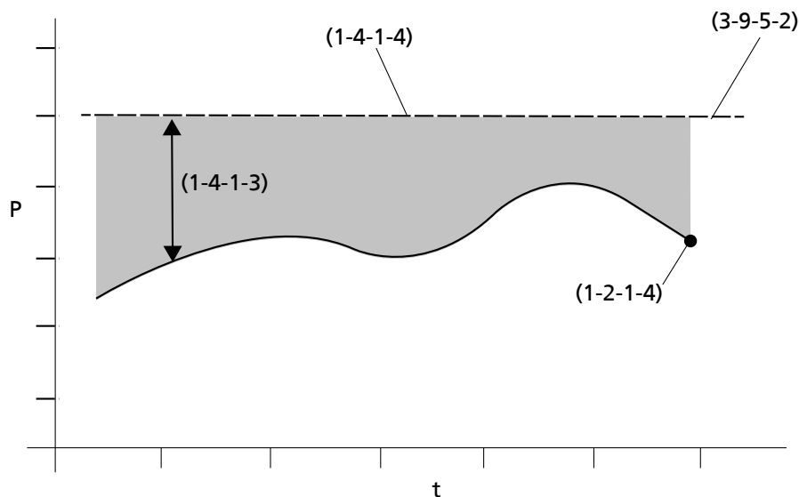
Рис. 79: Экономия электроэнергии с постоянной контрольной мощностью
