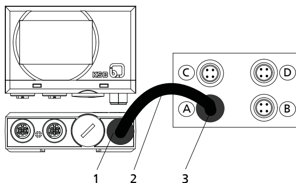
Рис. 37: Подключение PumpMeter к модулю M12 в одинарном режиме работы
