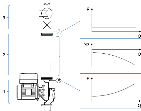
Рис. 71: Регулировка давления с подъемом зависящего от подачи заданного значения в открытой системе
