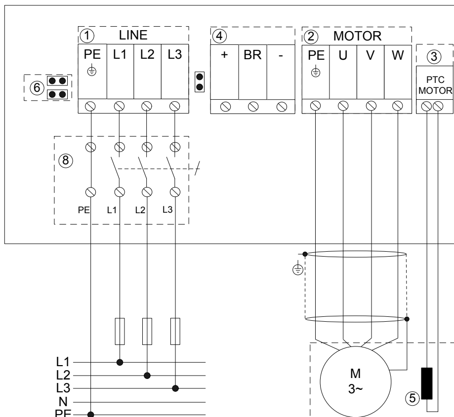
Рис. 21: Подключение кабеля электросети и двигателя к предусмотренным для этого клеммам, типоразмер D
