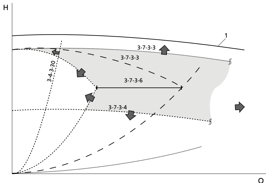
Рис. 66: Границы переключения двух работающих насосов в многонасосной системе
