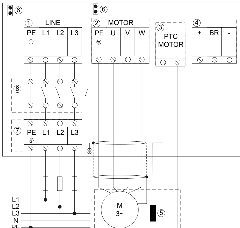
Рис. 20: Подключение кабеля электросети и двигателя к предусмотренным для этого клеммам, типоразмер В
