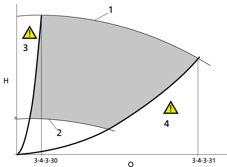
Рис. 69: График зависимости напора и подачи
