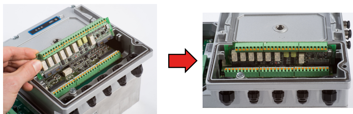
Рис. 45: Монтаж платы расширения ввода-вывода
