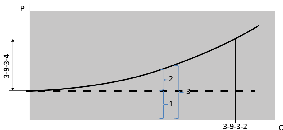
Рис. 73: Кривая изменения повышенного заданного значения при регулировании DFS на основе подачи
