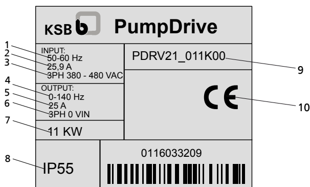
Рис. 6: Заводская табличка 1 – преобразователь частоты (пример)
