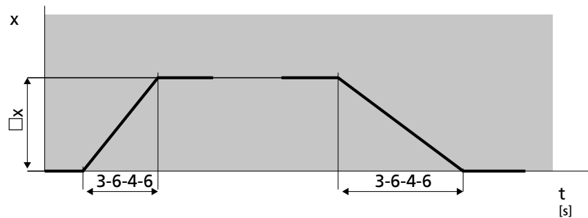
Рис. 84: Линейный сигнал заданного значения
