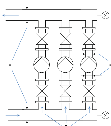
Рис. 70: Условия увеличения точности с помощью датчиков давления, установленных рядом с насосом, для многонасосных систем
