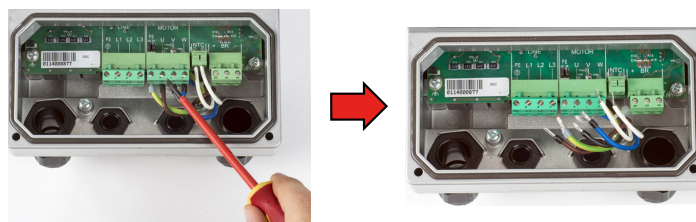
Рис. 22: Отсоединение жил разъема двигателя
