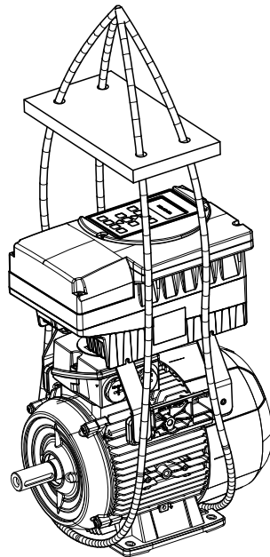
Рис. 4: Транспортировка двигателя с частотным преобразователем
