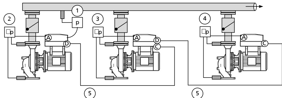
Рис. 90: Показания PumpMeter каждого насоса используются в качестве внутренней измеряемой величины, внешний датчик давления в качестве источника фактического значения.
