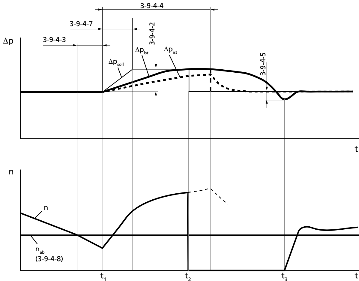
Рис. 78: Режим готовности с повышением заданного значения (здесь в качестве примера, после падения частоты вращения ниже значения отключения)
