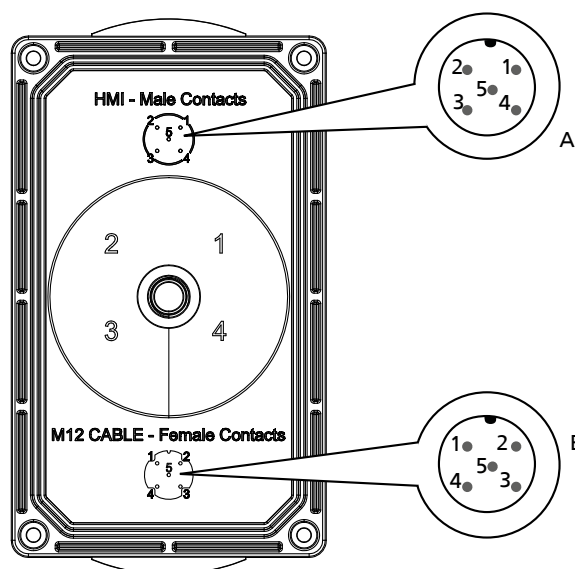
Рис. 53: Назначение выводов соединительного кабеля M12 и панели управления
