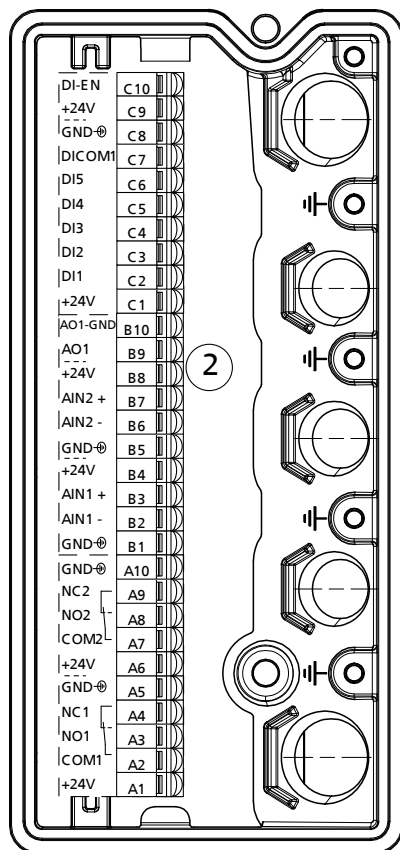
Рис. 51: Клеммы управления
