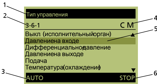
Рис. 56: Индикация меню
