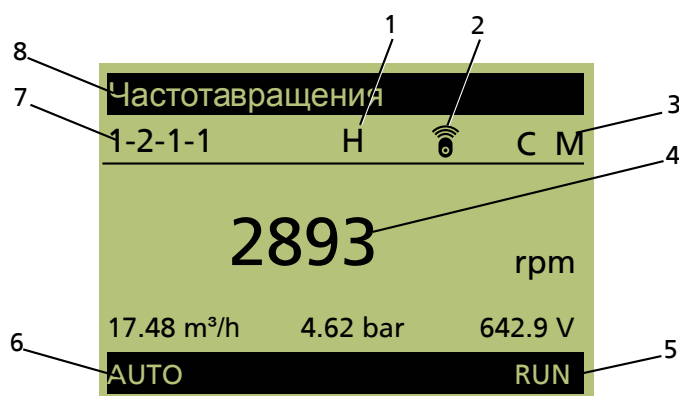
Рис. 55: Главный экран (пример)
