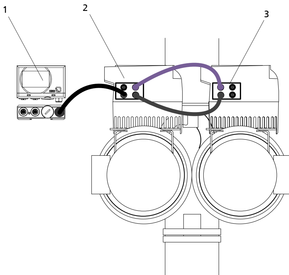
Рис. 91: PumpMeter как ведущее устройство Modbus
