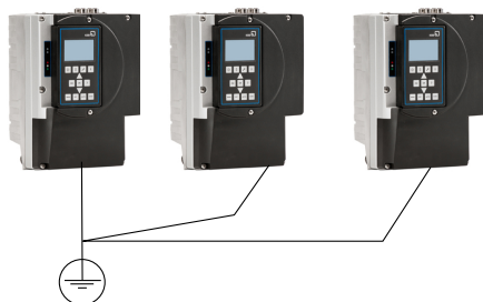
Рис. 31: Подключение заземления
