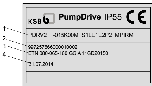
Рис. 7: Заводская табличка 2 – преобразователь частоты (пример)
