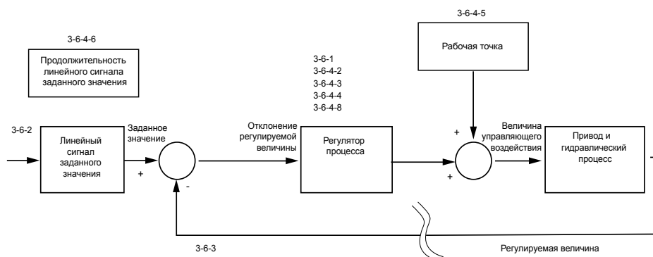
Рис. 62: Общая структура регулятора процесса
