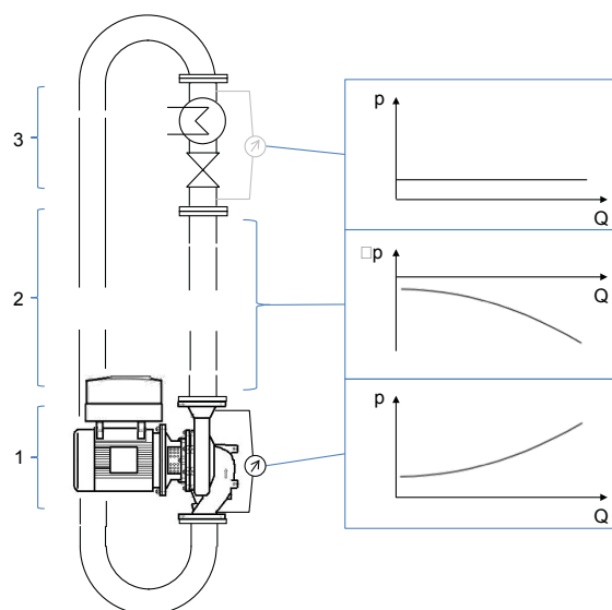
Рис. 72: Регулировка дифференциального давления с подъемом зависящего от подачи заданного значения в закрытой системе
