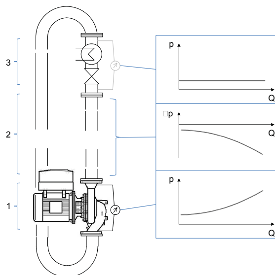
Рис. 76: Регулирование дифференциального давления с зависящим от подачи подъемом заданного значения в закрытой системе
