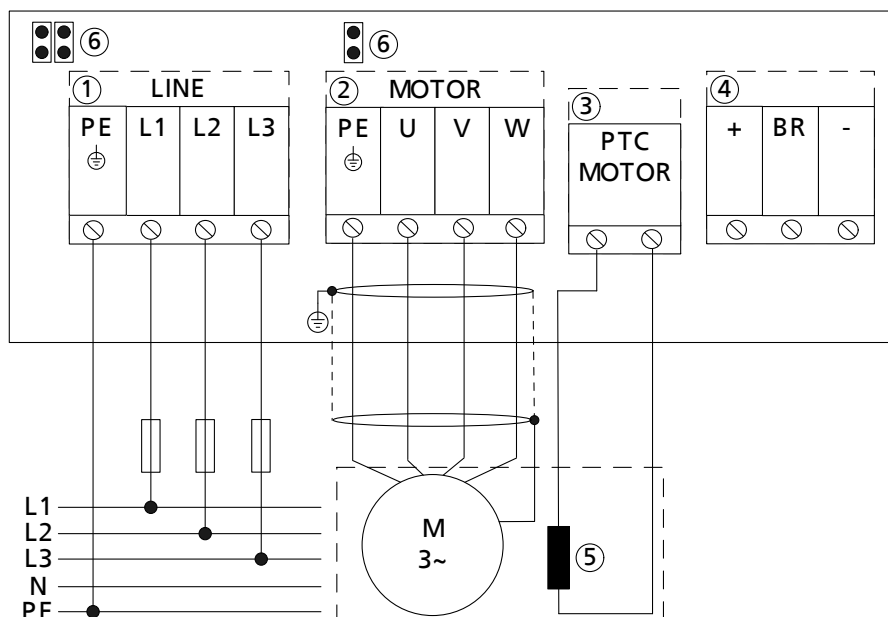
Рис. 15: Подключение к сети питания и двигателю, типоразмер А, исполнение 400 В/3 фазы
