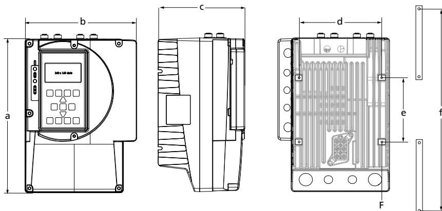
Рис. 8: Размеры
