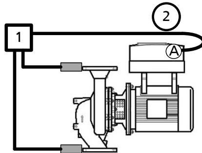
Рис. 89: PumpMeter в качестве источника фактического значения по шине Modbus
