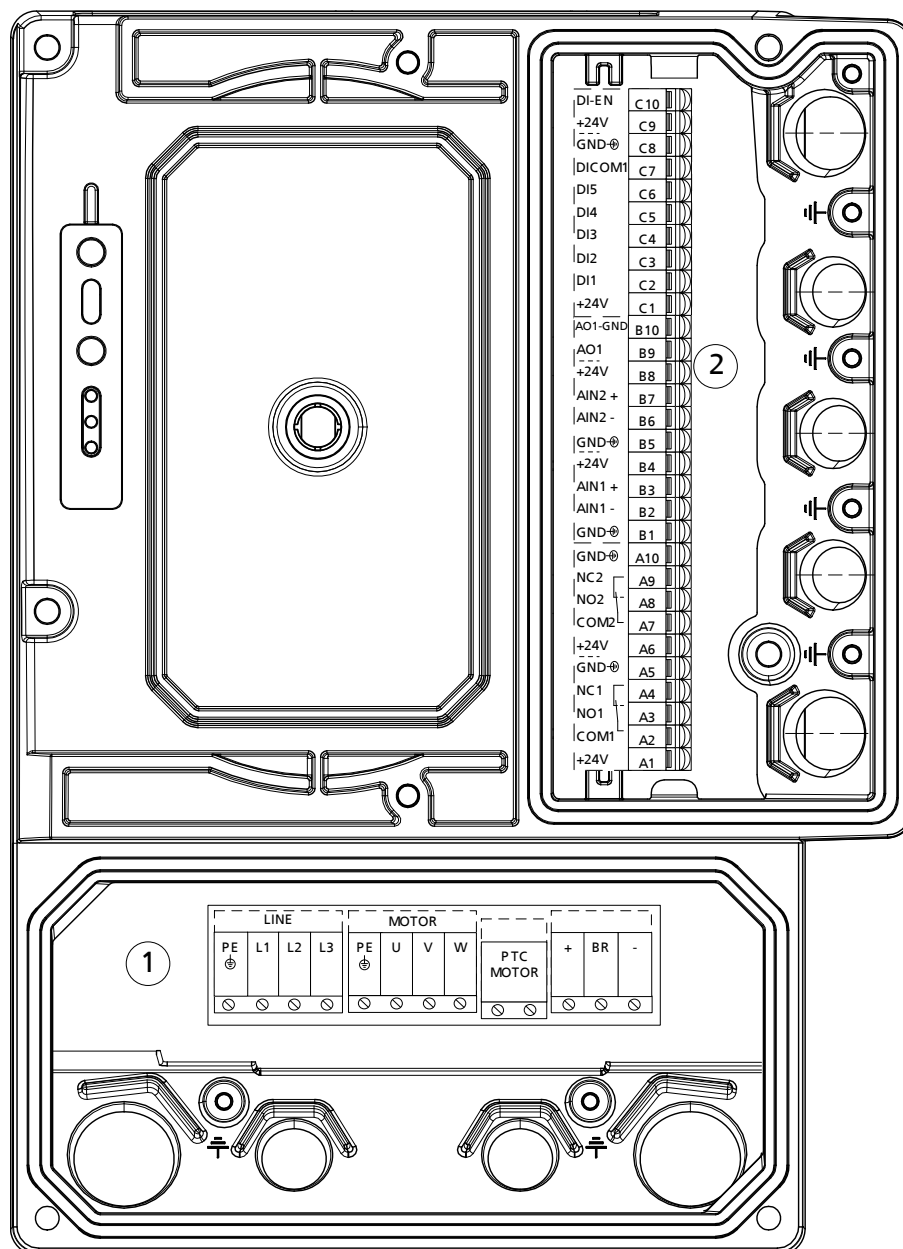
Рис. 14: Обзор клеммных колодок
