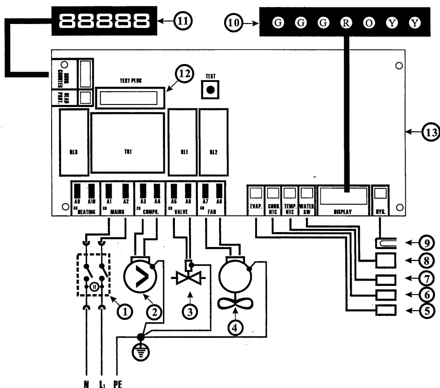
Схема электрических соединений
