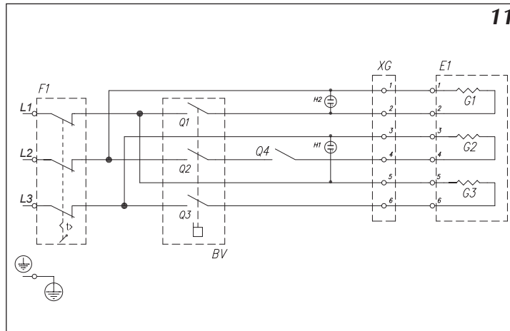
Рис.11 Принципиальная схема
