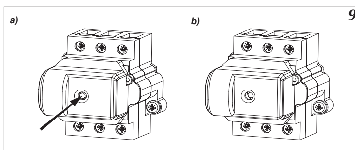
Рис.9 Выключатель по давлению WC-3
