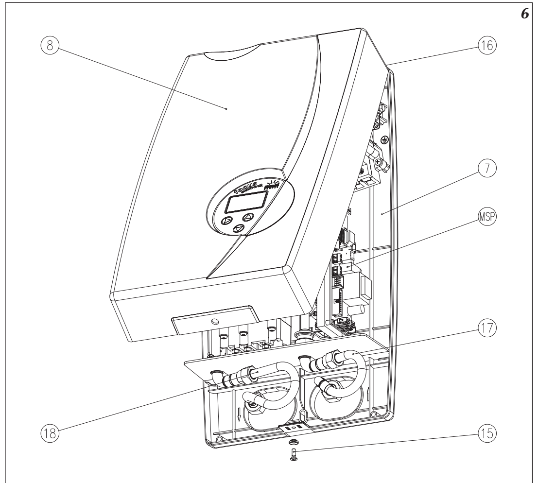
Рис.6 Внешний вид водонагревателя
