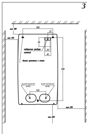
Рис.3 Монтажные условия
