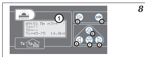
Рис.8 Панель управления ЕКСО.М1з/ ЕКСО.ТМ 1 - дисплей, 2-7 - клавиатура
