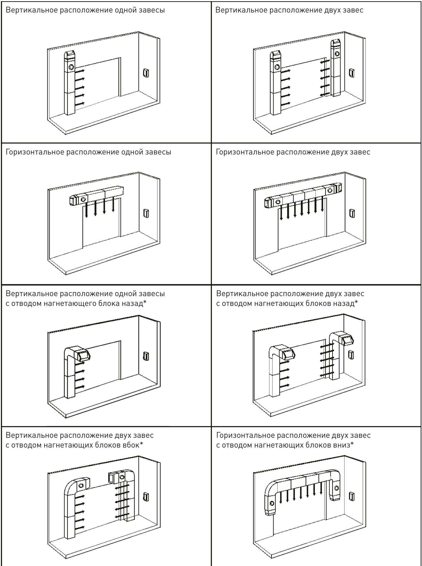
Рисунок 10. Варианты монтажа завес на дверном проеме
