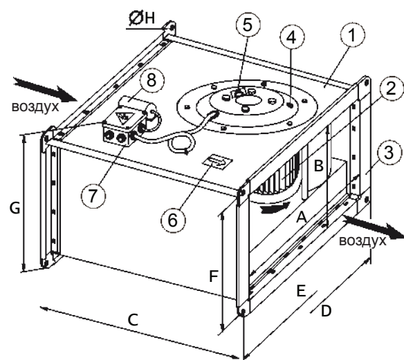
Рисунок 3. Устройство вентилятора
