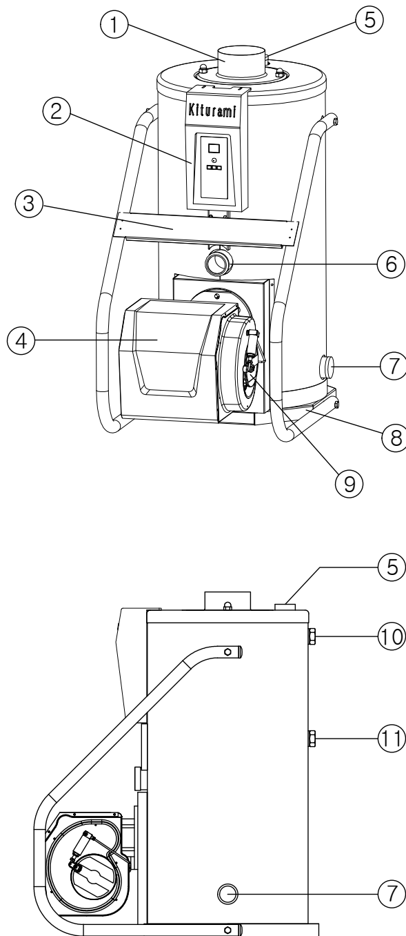
Рисунок 1. Устройство и назначение основных частей для котлов KSO HI FIN- 50/70/100
