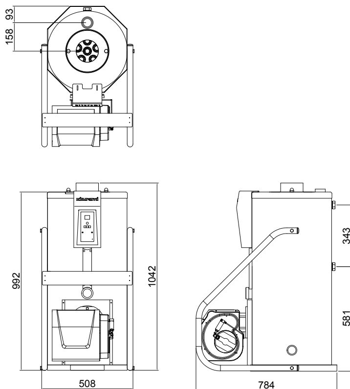
Рисунок 18. Габаритные и присоединительные размеры котлов KSO HI FIN-70
