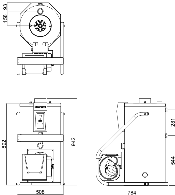
Рисунок 17. Габаритные и присоединительные размеры для котлов KSO HI FIN-50
