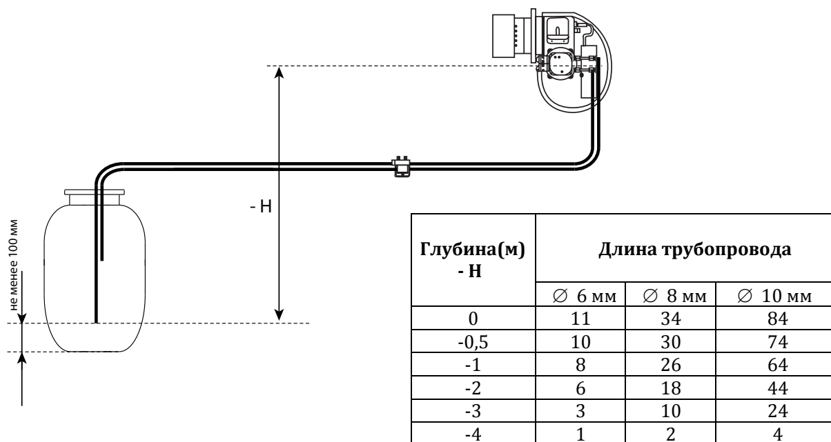
Подключение горелки в случае размещения топливного бака ниже котла.
