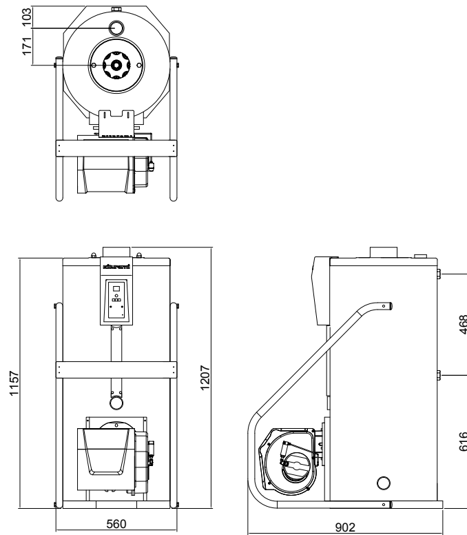
Рисунок 19. Габаритные и присоединительные размеры котлов KSO HI FIN-100
