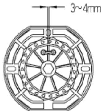
Рисунок 21. Схема регулировки системы поджига
