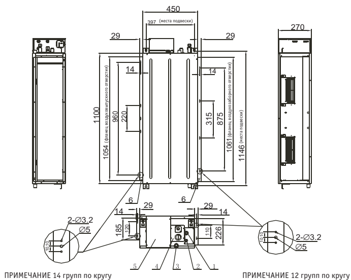
Рис. 8 (только для моделей серии KSTV70HFAN1)
