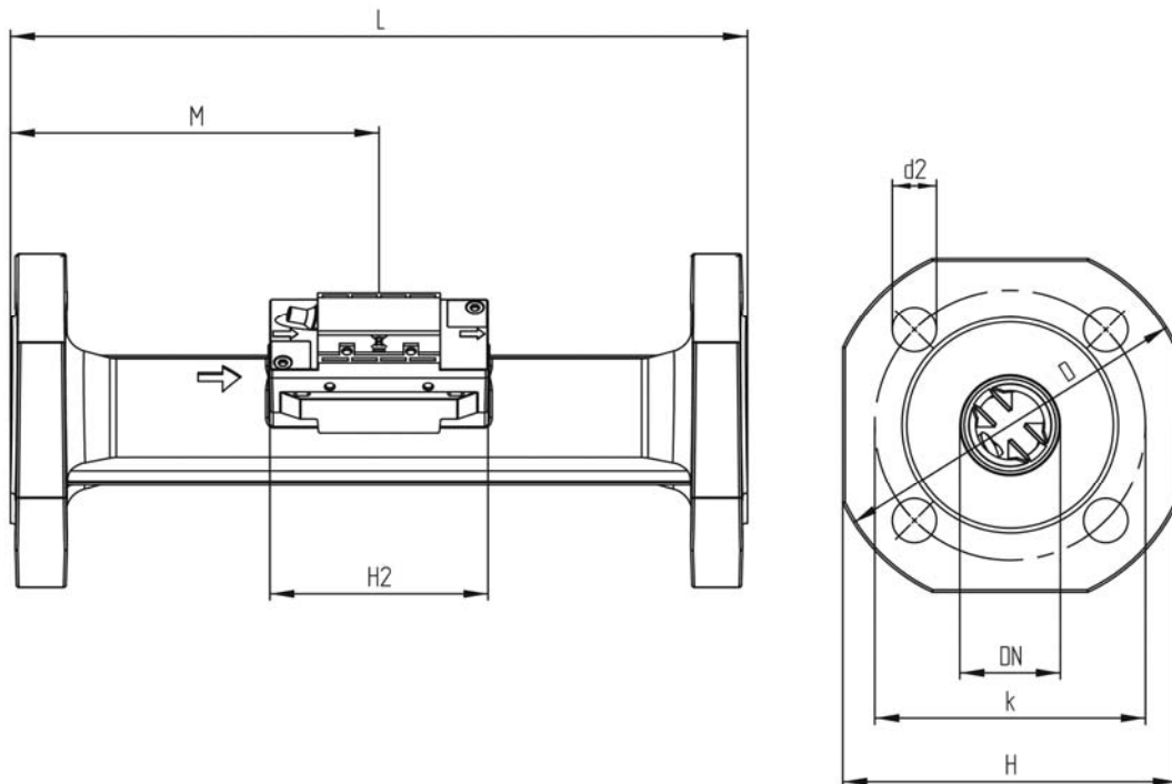
Рис. 5: Расходомер с фланцевым присоединением Ду25 - Ду50
