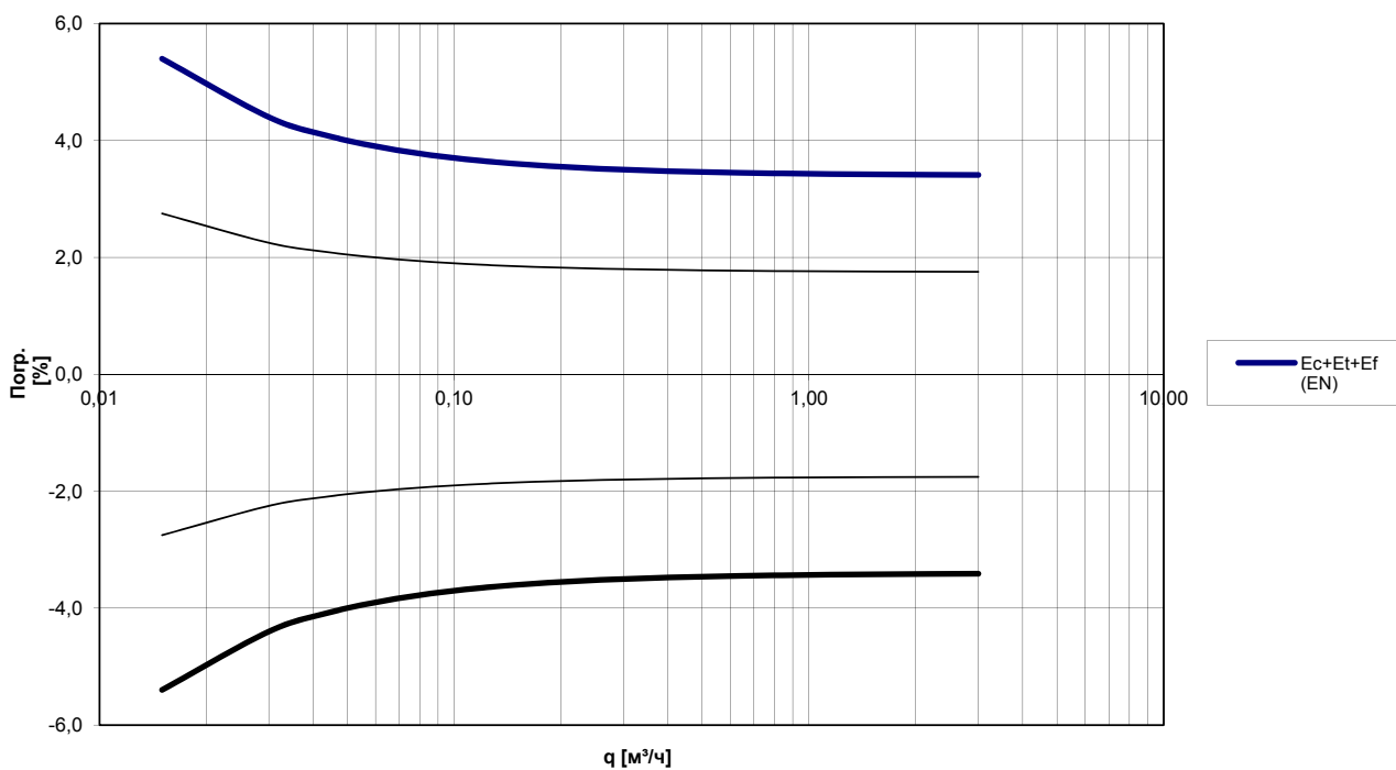
График 1: Типичная точность MULTICAL® 402 в сравнении с требованиями EN 1434
