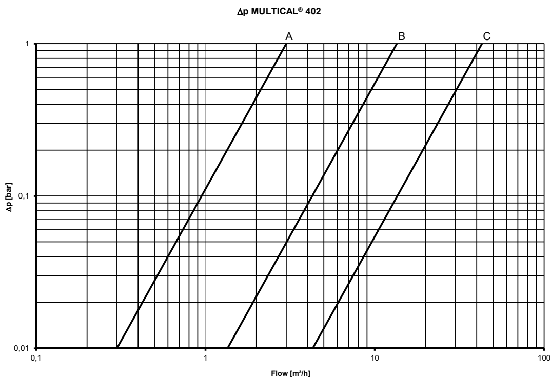
График 2 Потери давления
