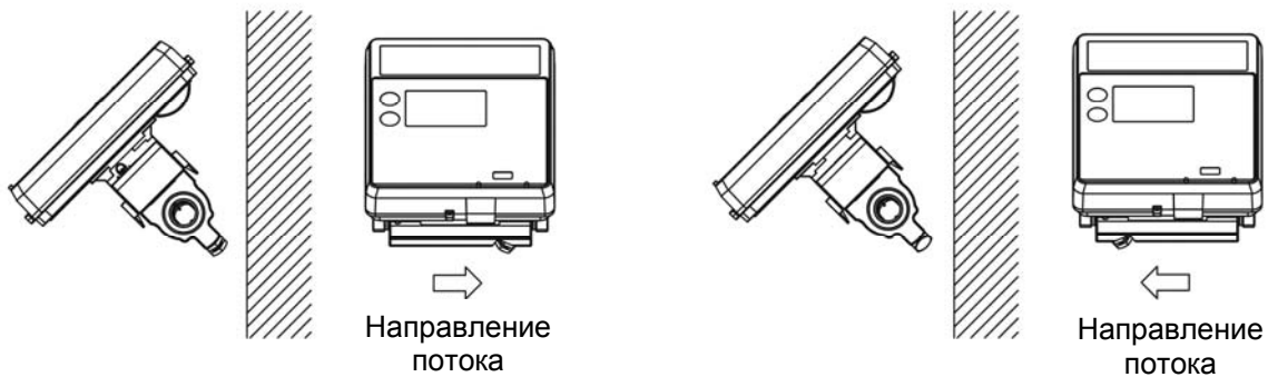
Рис. 11: Монтаж счетчика с резьбовым присоединением
