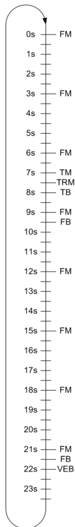
Нормальный цикл (24 с)
