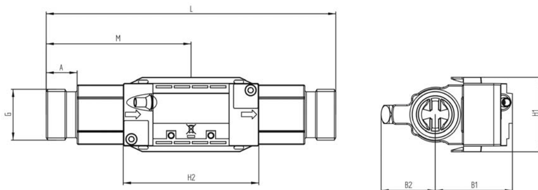
Рис. 3: Расходомер с резьбовым присоединением G¾ и G1
