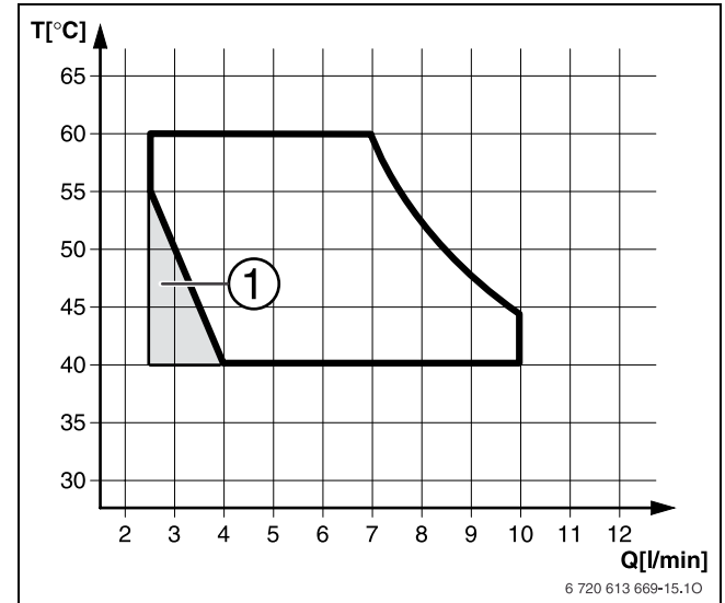
Рис 24 Диаграмма при температуре холодной воды на входе +10 °С
