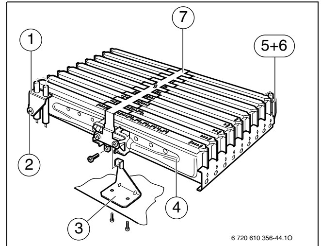
Рис 37 Узел горелки
