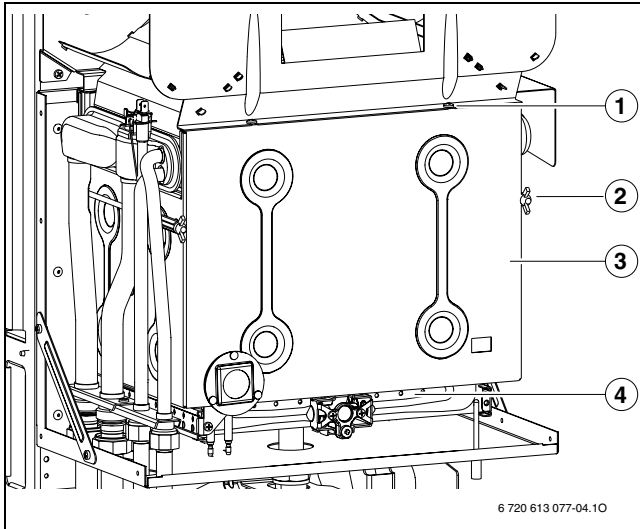
Рис 36 Открывание горелки
