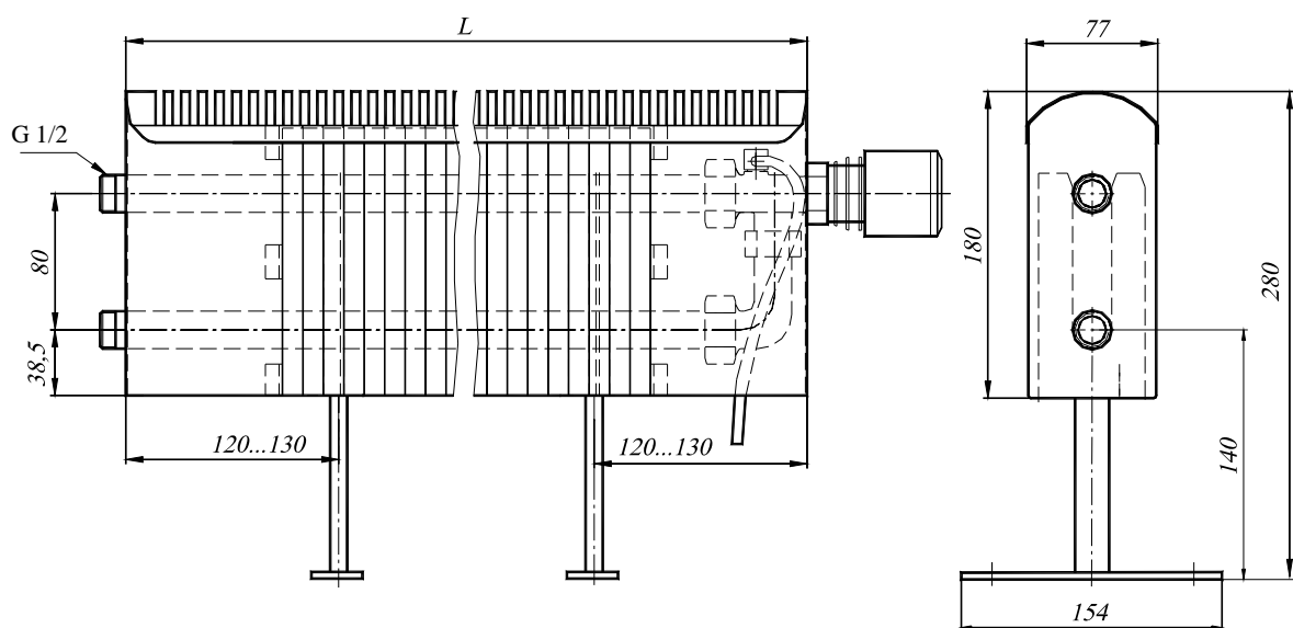
Рис. 1.29. Конвектор «НовоТерм» напольный концевой SKO 200 T16 с терморегулирующим клапаном для однотрубных систем отопления и встроенным замыкающим участком.
