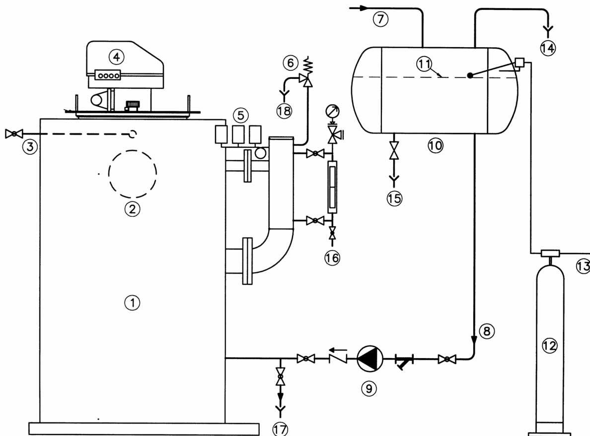
Рис. 8 – Схема установки
