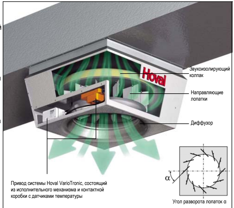
Рис. 1 Воздухораспределитель Hoval Air-Injector
