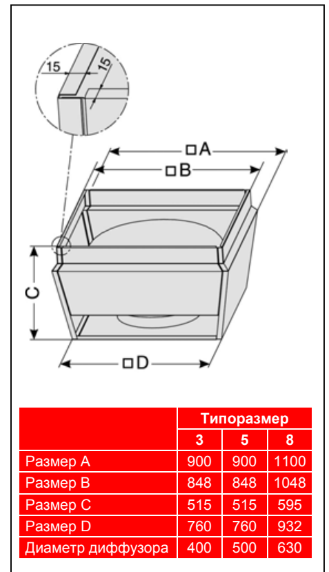
Рис. 3. Габаритные размеры агрегата, мм
