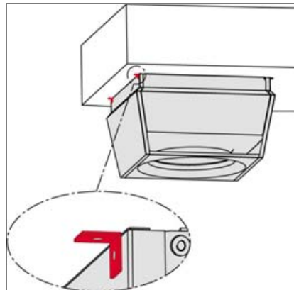
Рис. 2. Пример монтажа
