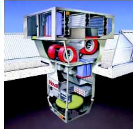
Приточно-вытяжной агрегат без рекуперации тепла - LH
