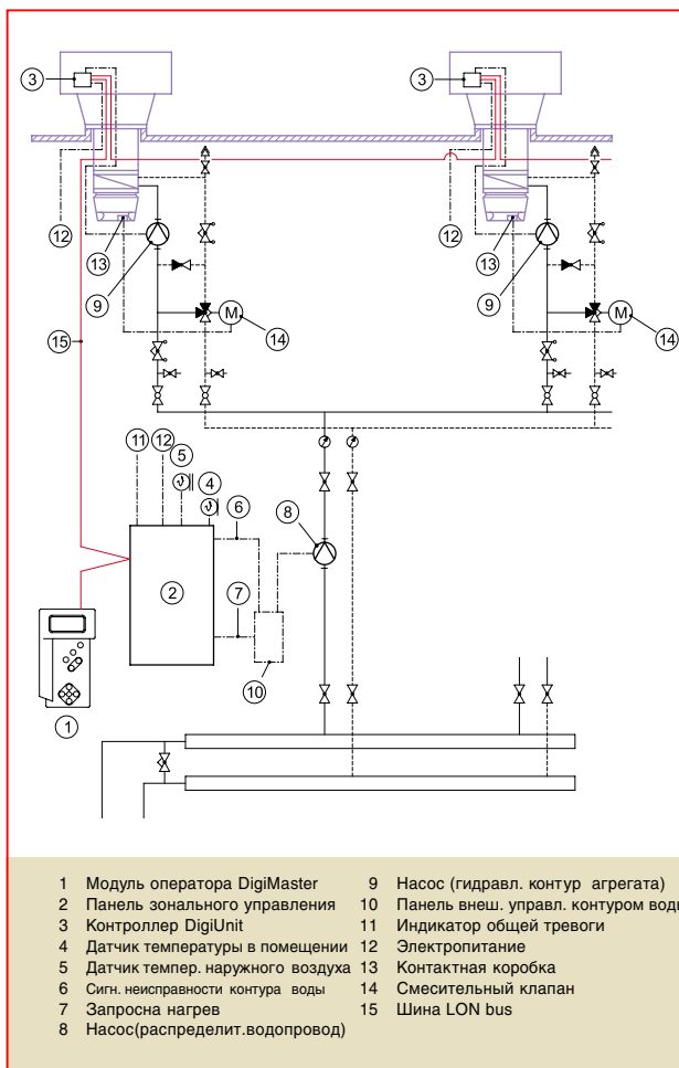
Рис. В-4: Гидравлическая система инъекционного типа
