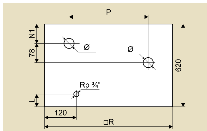
Рис. 16: Размеры секции воздухоохладителя
