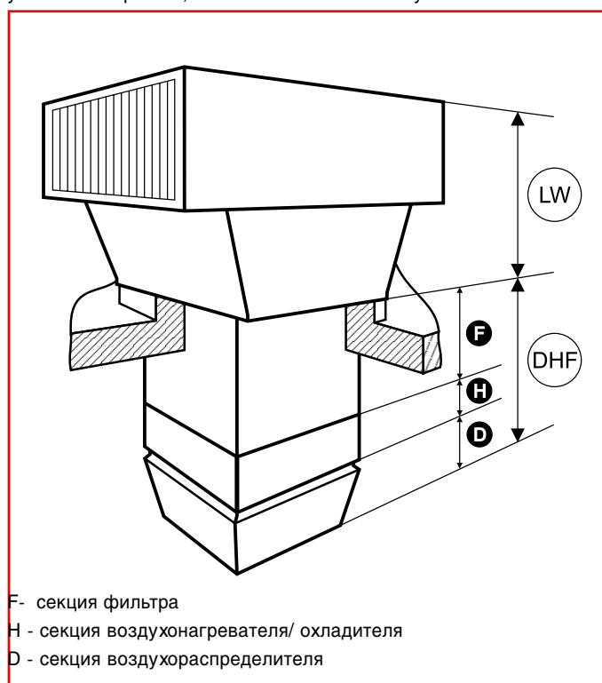
Рис. 1: Основные секции агрегата LHW
