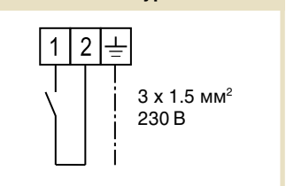
Рис. 22: Схема электроподключения
