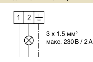
Рис. 23: Схема электроподключения
