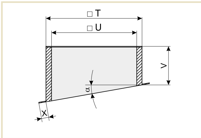
Рис. 10: Указываемые в заказе размеры для монтажного основания с вертикальными стенками (DG)
