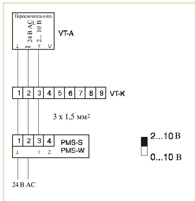
Рис. А-3: Электросхема подключения потенциометра для управления воздухом распределителем
