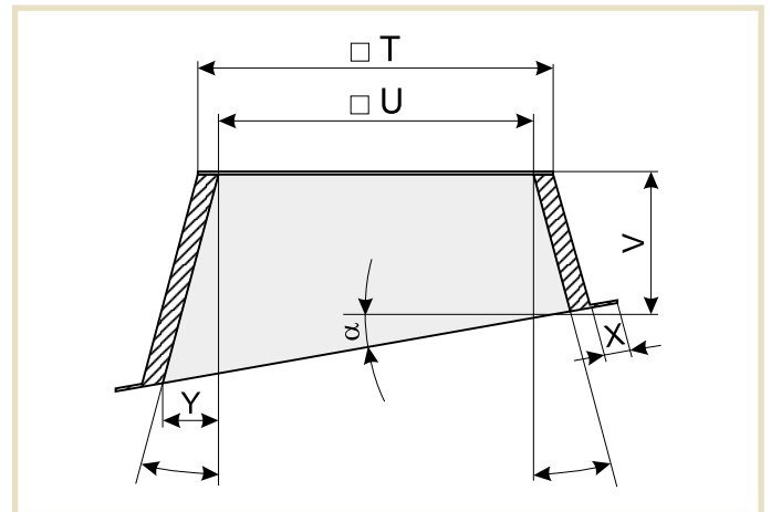
Рис. 12: Указываемые в заказе размеры для монтажного основания с коническими стенками (DK)
