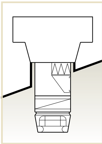
Рис. 9: Монтажное основание с вертикальными стенками
