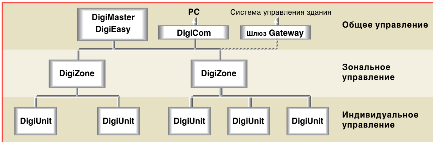
Рис. 17: 3 иерархических уровня управления системы Noval DigiNet
