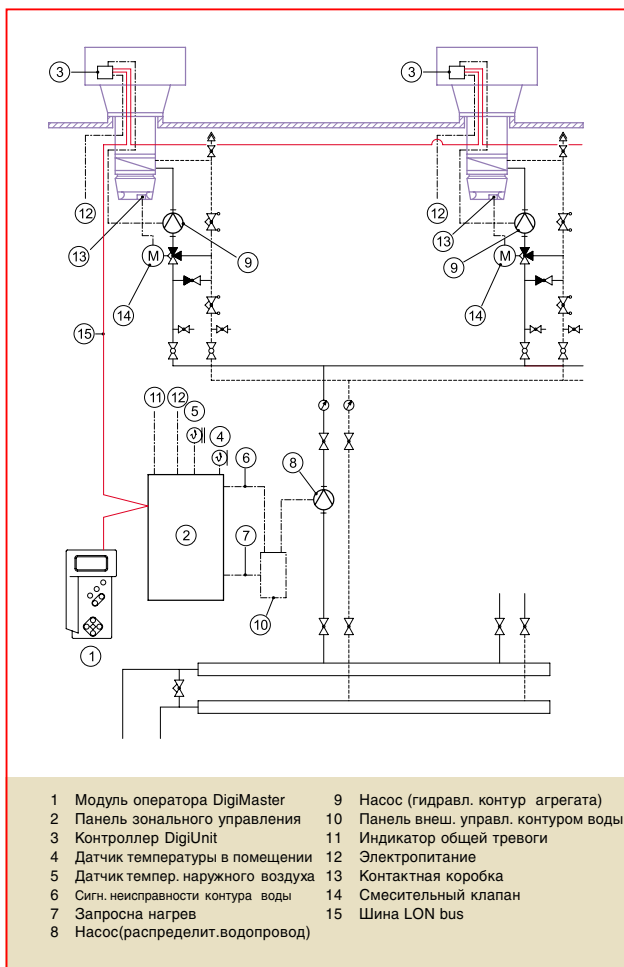
Рис. В-3: Гидравлическая система смесительного типа
