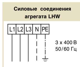
Рис. 24: Силовые соединения агрегата LHW
