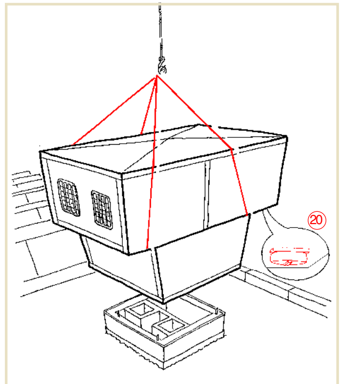
Рис. 34: Нижний и верхний блоки должны быть правильно ориентированы по отношению друг к другу
