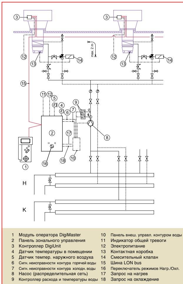
Рис. С-3: 2-х трубная гидравлическая система (Пример: девиационная система)
