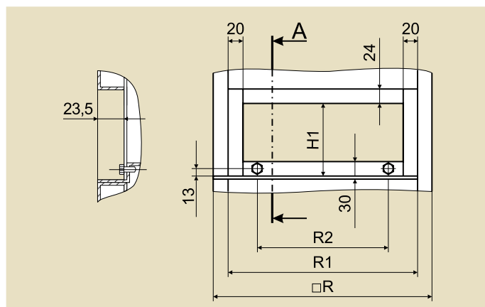
Рис. 14: Размеры фланца в секции фильтра для подсоединения вытяжного воздуховода
