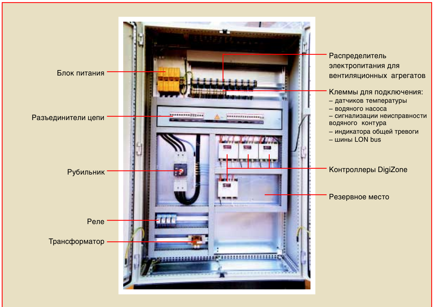
Рис. 20: Внутренние компоненты панели зонального управления
