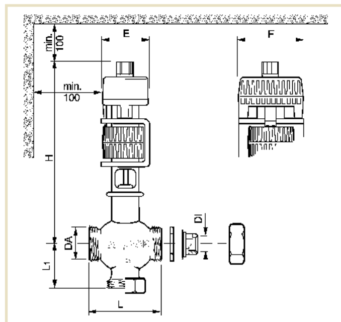
Рис. 13: Стандартный смесительный клапан
