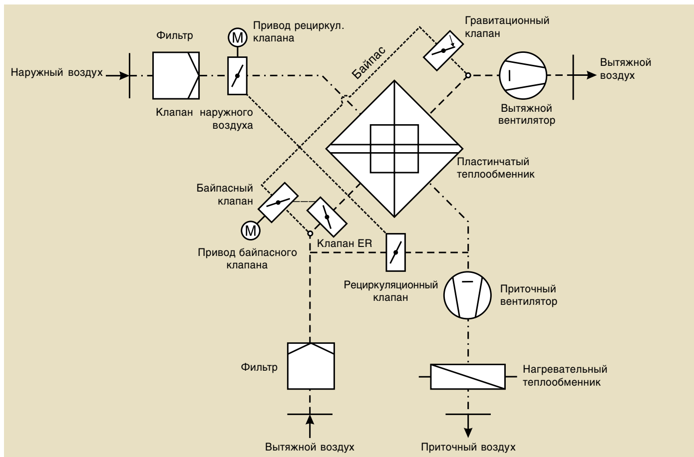
Рис. 3: Схема распределения воздушных потоков
