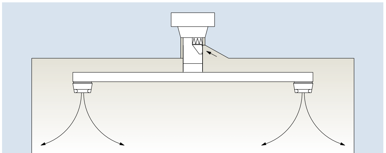
Устройство приточного воздуховода с двумя подсоединенными воздухораспределителями
