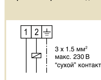
Рис. 21: Схема электроподключения
