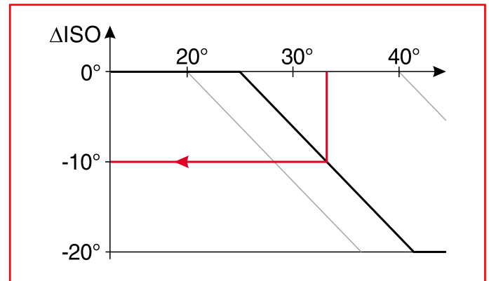
График А-3: Поправка для летнего режима ("Int_Point_Shift")
