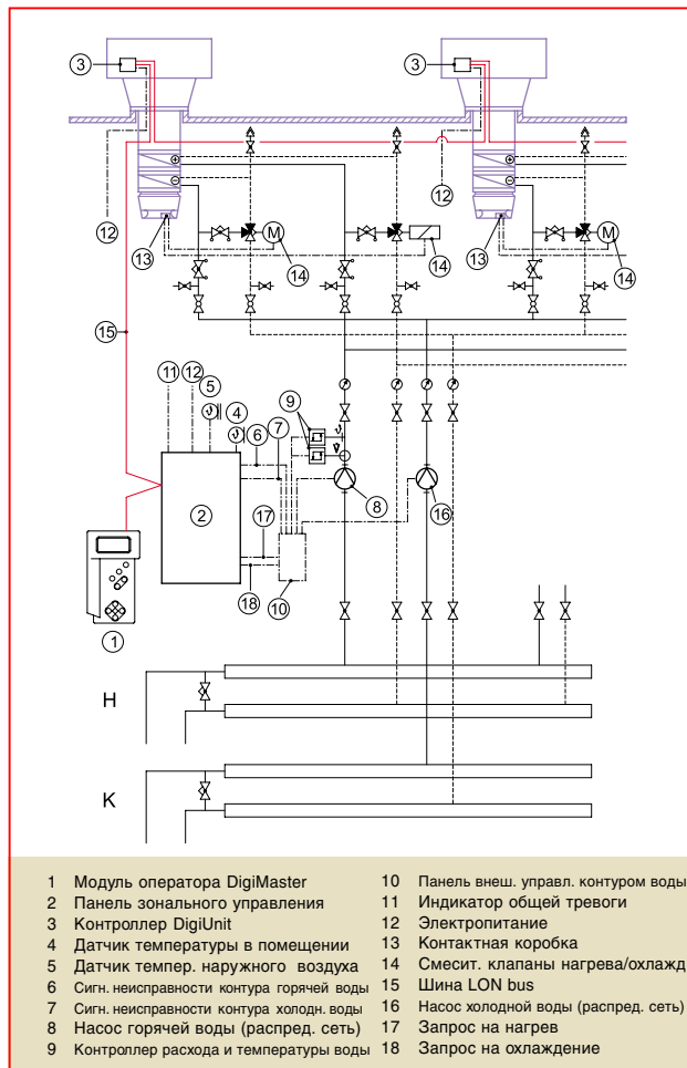
Рис. С-4: 4-х трубная гидравлическая система (Пример: девиационная система)
