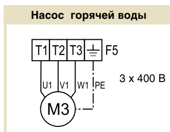
Рис. В-1: Схема подключения насоса горячей воды
