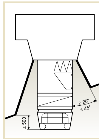
Рис. 11: Монтажное основание с коническими стенками
