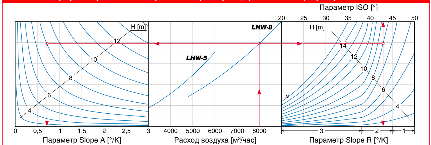
График А-4: График определения настроечных параметров управления воздухораспределением
