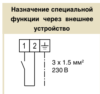
Рис. 26: Схема электроподключения контактов панели управления к внешнему устройству
