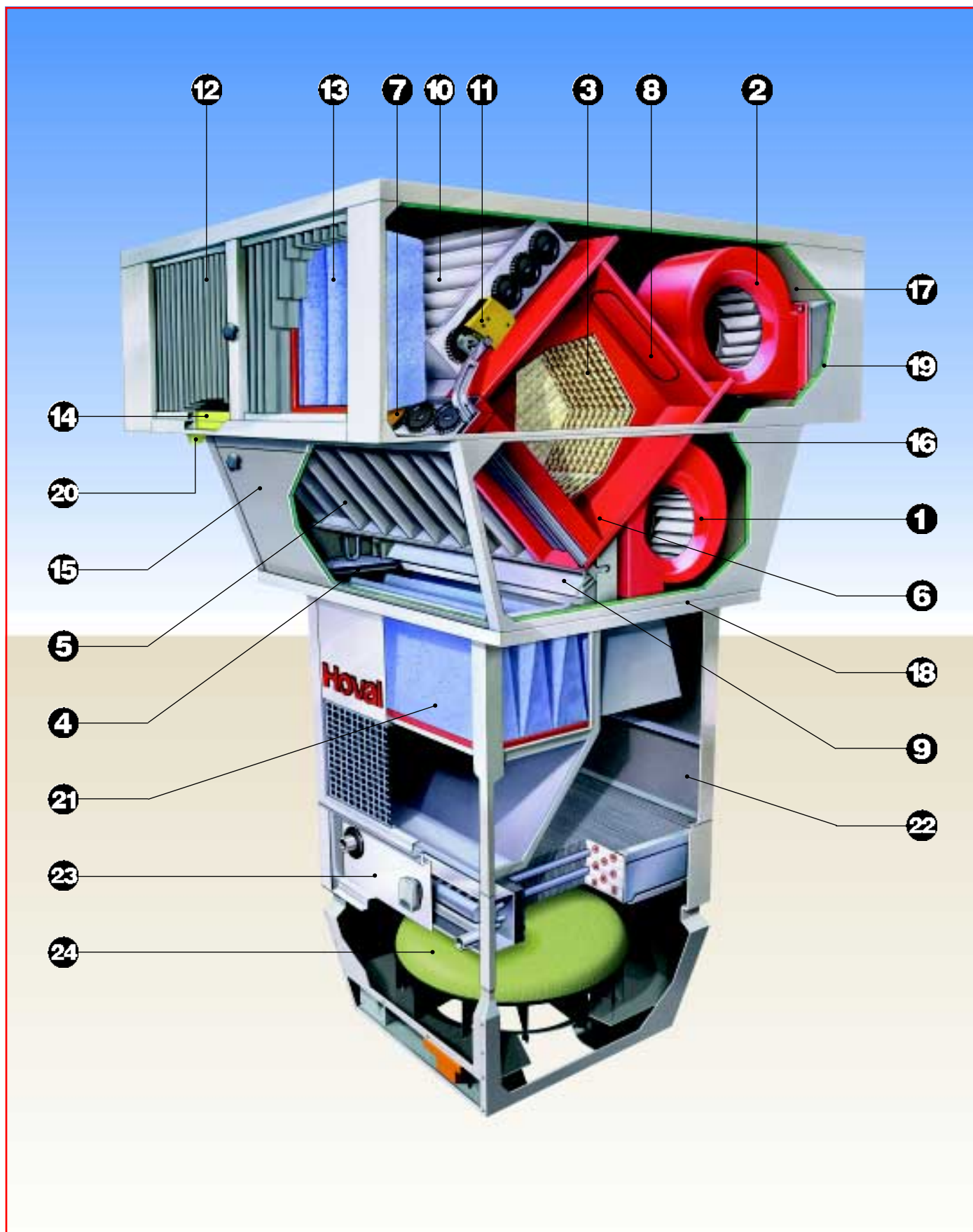
Рис. 2: Конструкция агрегата LHW
