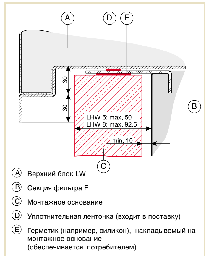
Рис. 8: Совмещение верхнего и нижнего блоков с монтажным основанием
