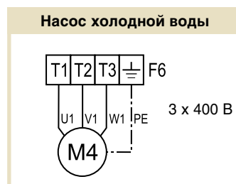
Рис. В-2: Схема подключения насоса холодной воды
