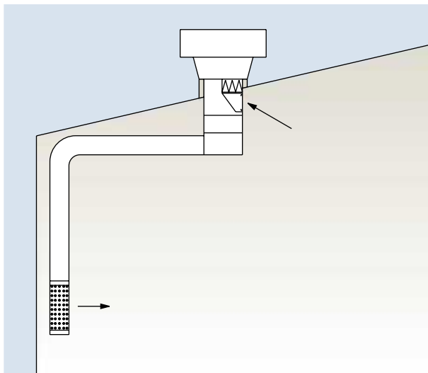
Организация притока в нижнюю зону помещения
