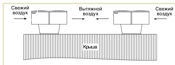
Рис. 27: Расположение агрегатов с выходными отверстиями напротив друг друга
