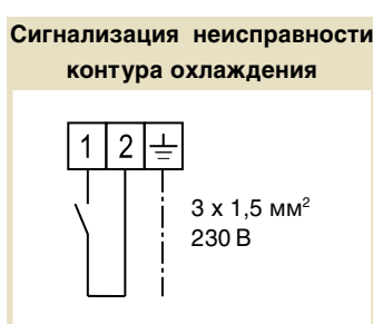
Рис. С-2: Электросхема подключения
