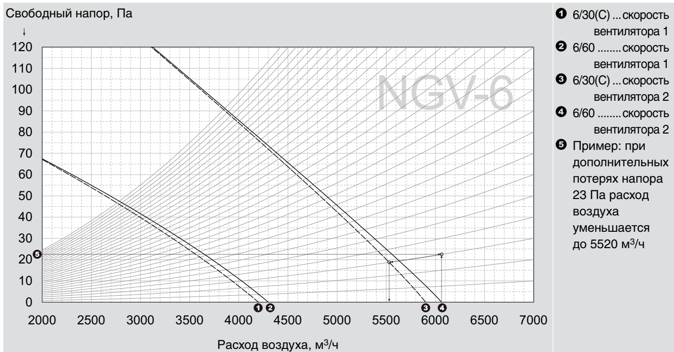
График С3-1. Расход воздуха для агрегата TopVent® NGV-6 при свободном напоре
