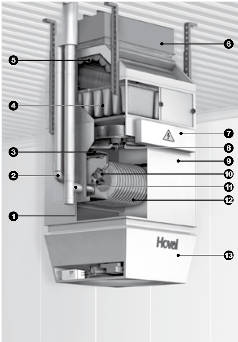
Рис. E2-2. Конструкция агрегата TopVent® MG
