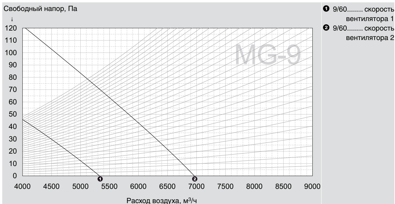
График ЕЗ-2. Расход воздуха для агрегата TopVent® MG-9 при дополнительных потерях напора
