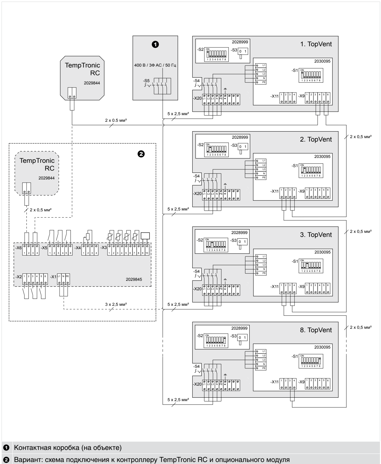
Рис. В7-2. Электросхема подключения агрегата TopVent® DGV
