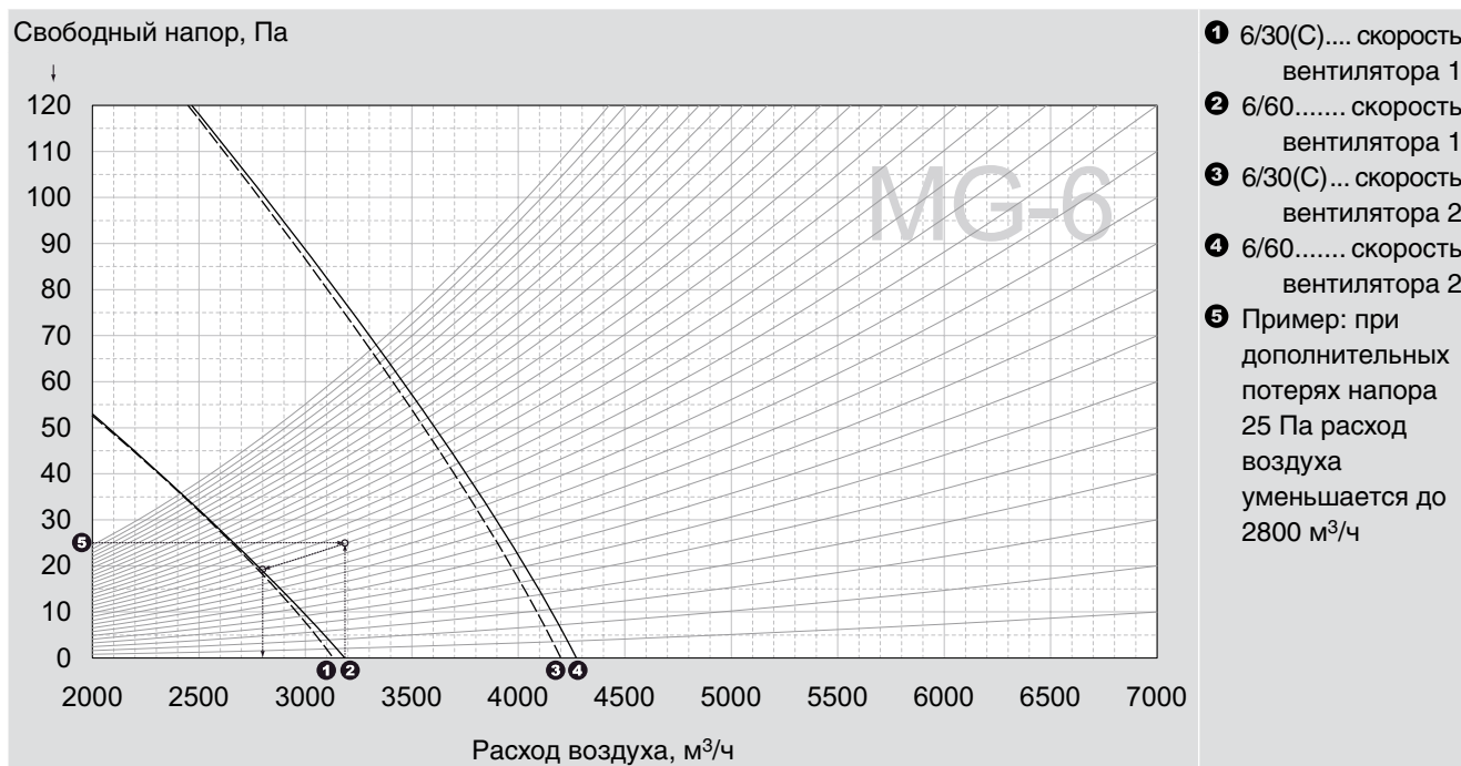
График ЕЗ-1. Расход воздуха для агрегата TopVent® MG-6 при дополнительных потерях напора
