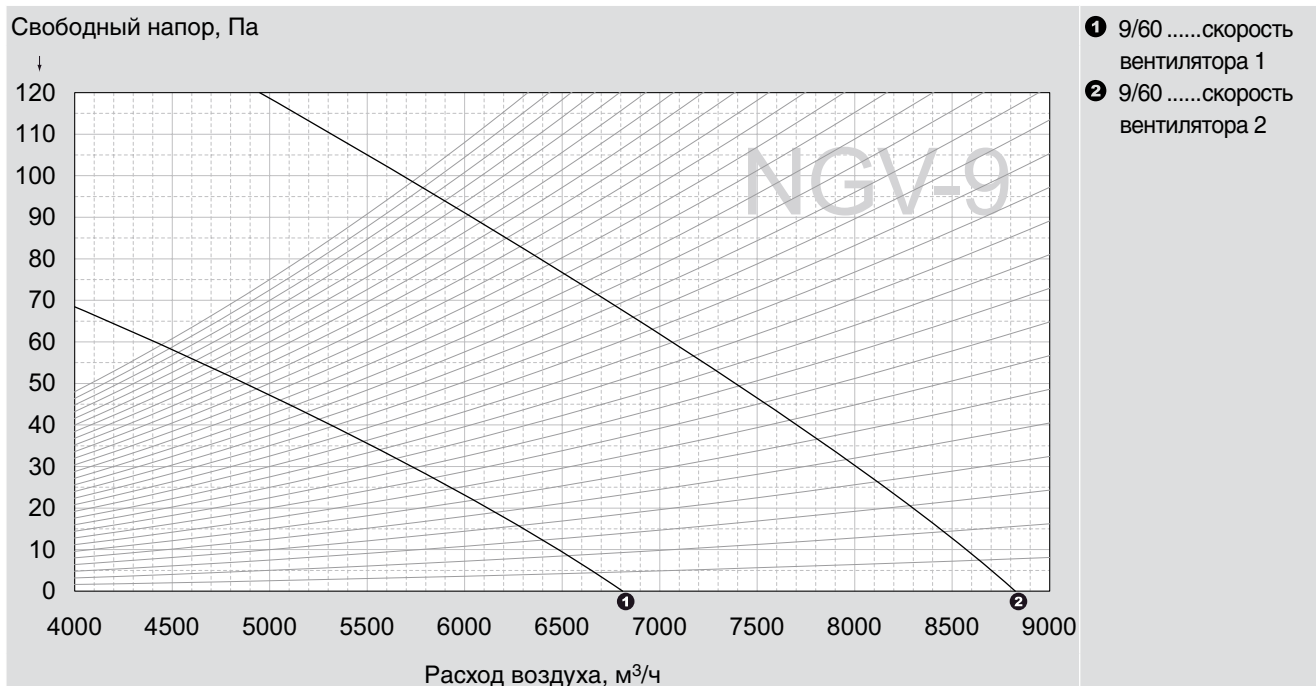
График С3-2. Расход воздуха для агрегата TopVent® NGV-9 при дополнительных потерях напора
