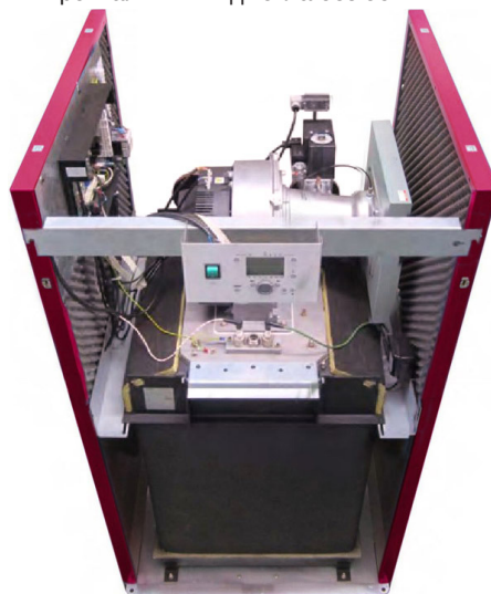
Фронтальный вид котла без обшивки
