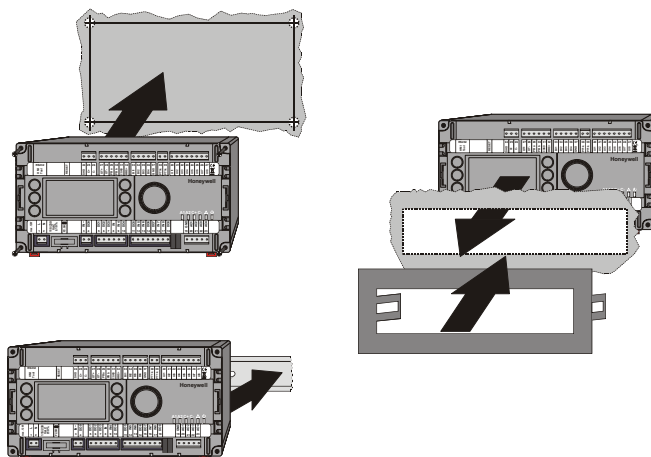
Рис. 3. Варианты монтажа
