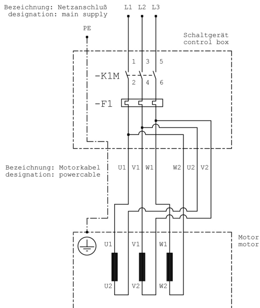
Abb. 4 / Fig. 4: Netzanschluss Direkt-Start (DOL) für Stern-Dreieck- vorbereite Motoren (Alle Wicklungsenden über Anschlusskabel zugänglich) Dreieckschaltung der Wicklung Starter Connection Direct-on-Line (DOL) Start for Star-Delta prepared Motors Delta Connection of Sta- tor Windings Netaansluiting Direkt-Start (DOL) voor Ster-Driehoek voorbereide motoren (Alle wikkeleingseinden met aansluitkabel toegankelijk) Driehoeksschakeling van de wikkeling
