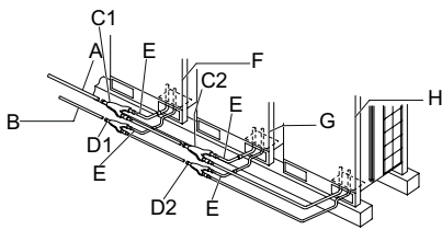
Подвод труб спереди или сзади
