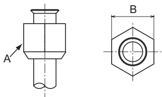
Расстояние -B- между гранями гайки -A-
