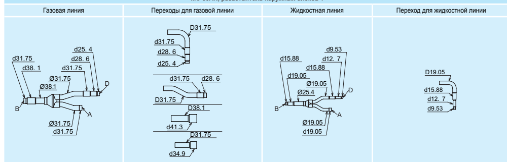
MC-30AN, разветвитель наружных блоков 1
