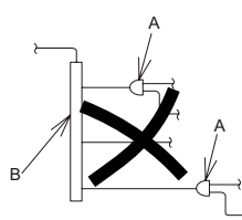
Рисунок 4. Не присоединяйте тройник к коллектору
