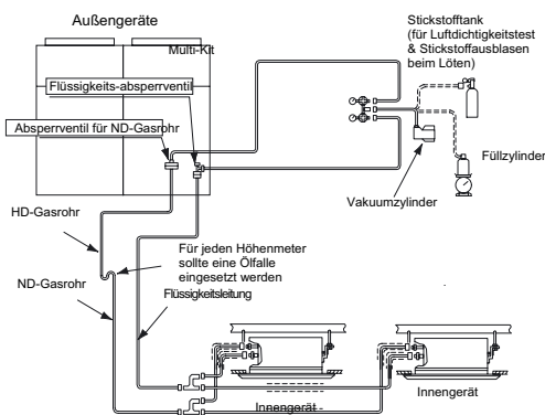
Beispiel einer Entleerung und Befüllung mit Kältemittel FSN
