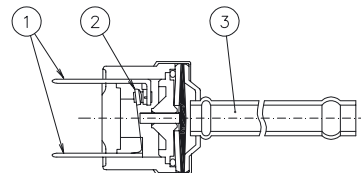
Struktur des Hochdruckschalters Pressure Switch
