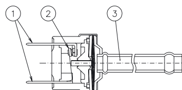
Struktur på højtryksafbryder
