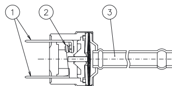
Structure du pressostat haute pression
