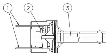
Estructura del preostato de alta presión
