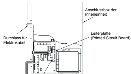
Anschluss für Automatik-Schwingmotor (Niederspannung 7-Pin ROT)
