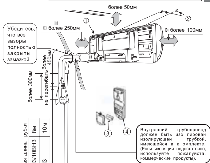
Рисунок, показывающий Монтаж ВНУТРЕННЕГО и НАРУЖНОГО БЛОКОВ
