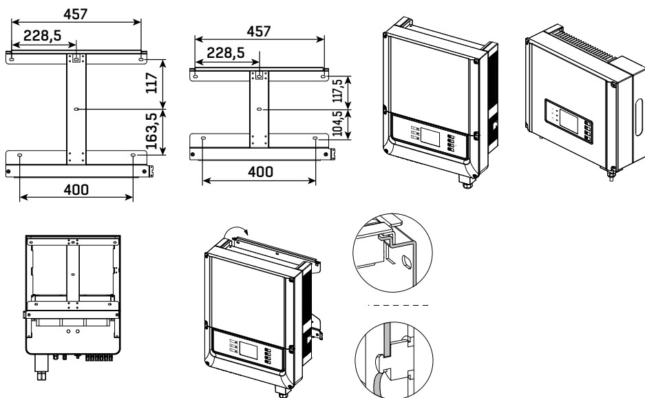
Рисунок 3.4.4 Инструкция по креплению инвертора на поверхность
