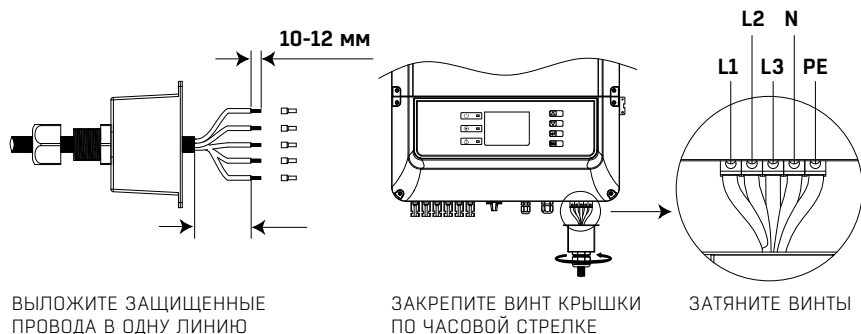
Рисунок 3.4.6 Подключение инвертора к сети
