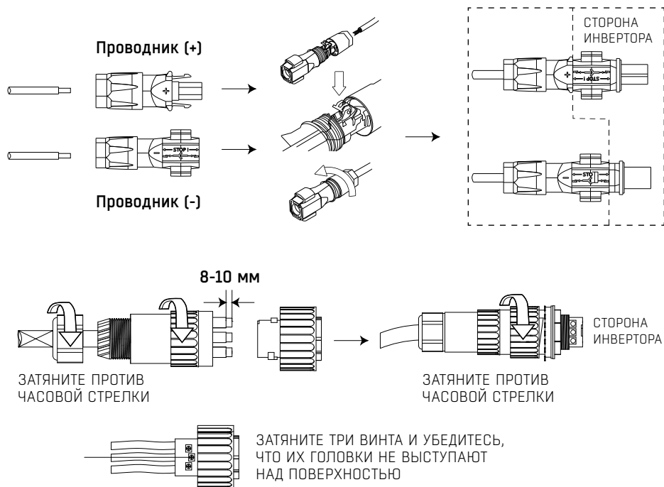
Рисунок 3.4.7 Инструкция по монтажу кабелей
