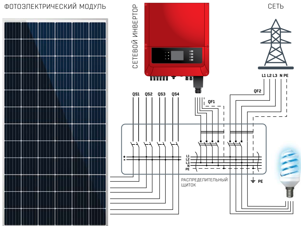
Блок-схема по подключению оборудования Системы С4-М
