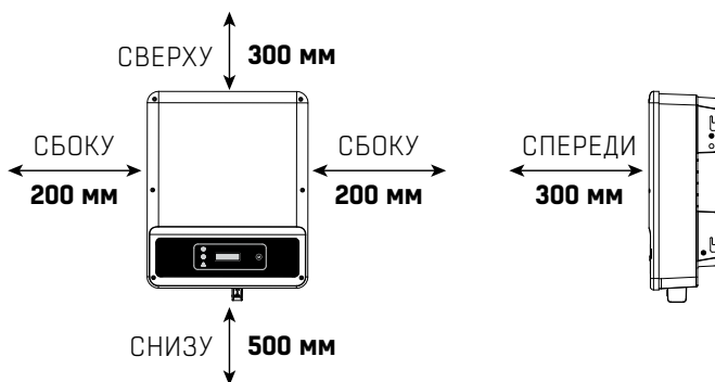
Рисунок 3.4.3 Расстояния до места установки инвертора
