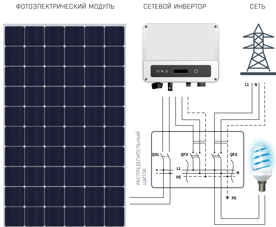
Блок-схема по подключению оборудования Системы СЗ
