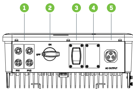
Рисунок 2.3.1 Схема инвертора
