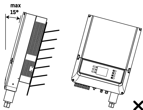
Рисунок 3.4.2 Установка инвертора на поверхность
