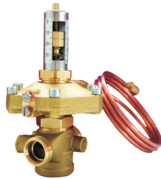
Регулятор перепада давления HERZ 4002
