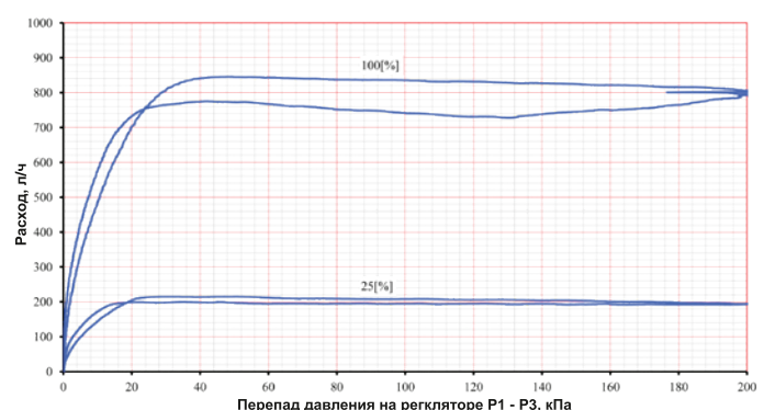
Гистерезис регулятора расхода 4001 (настройки: 25% и 100% максимального расхода)
