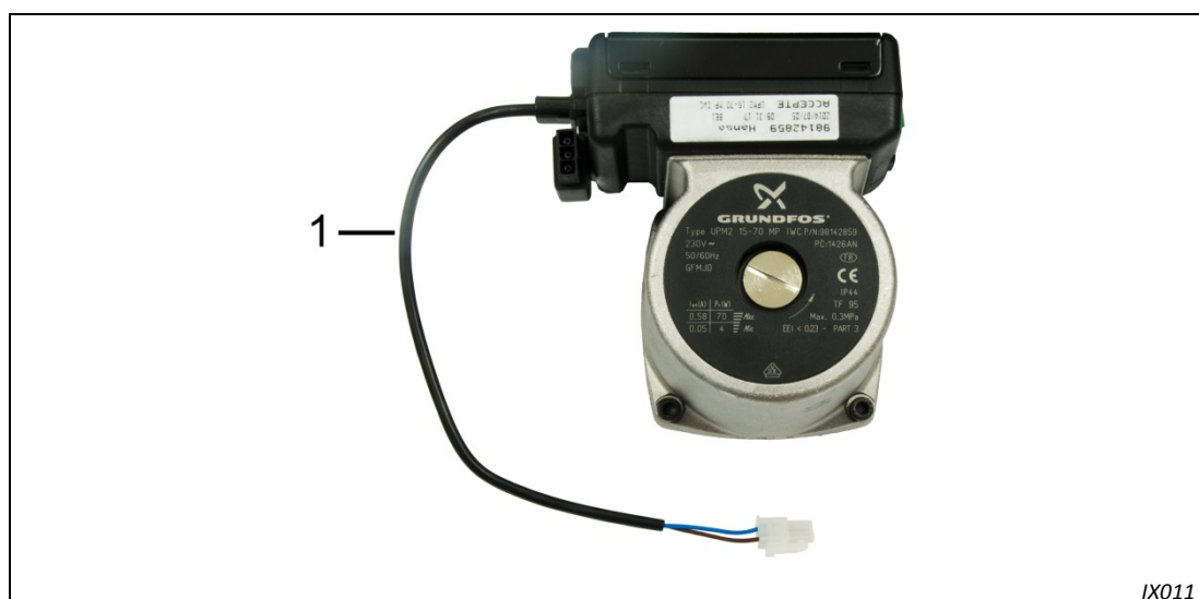
Рис. 14: Головка насоса
