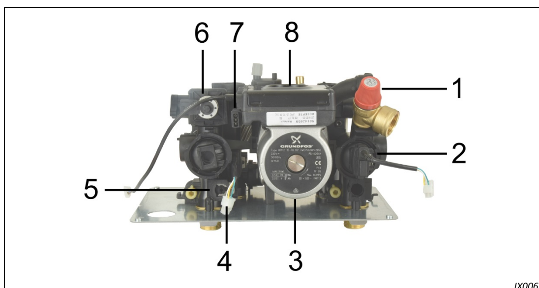
Рис. 11: Гидроблок UPS 15-60 MP IWC
