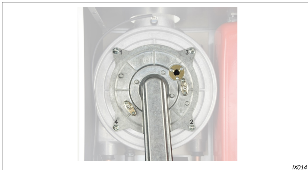
Рис. 27: Ослабление гаек
