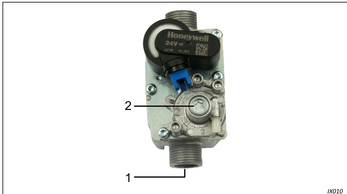
Рис. 12: Газовый клапан
