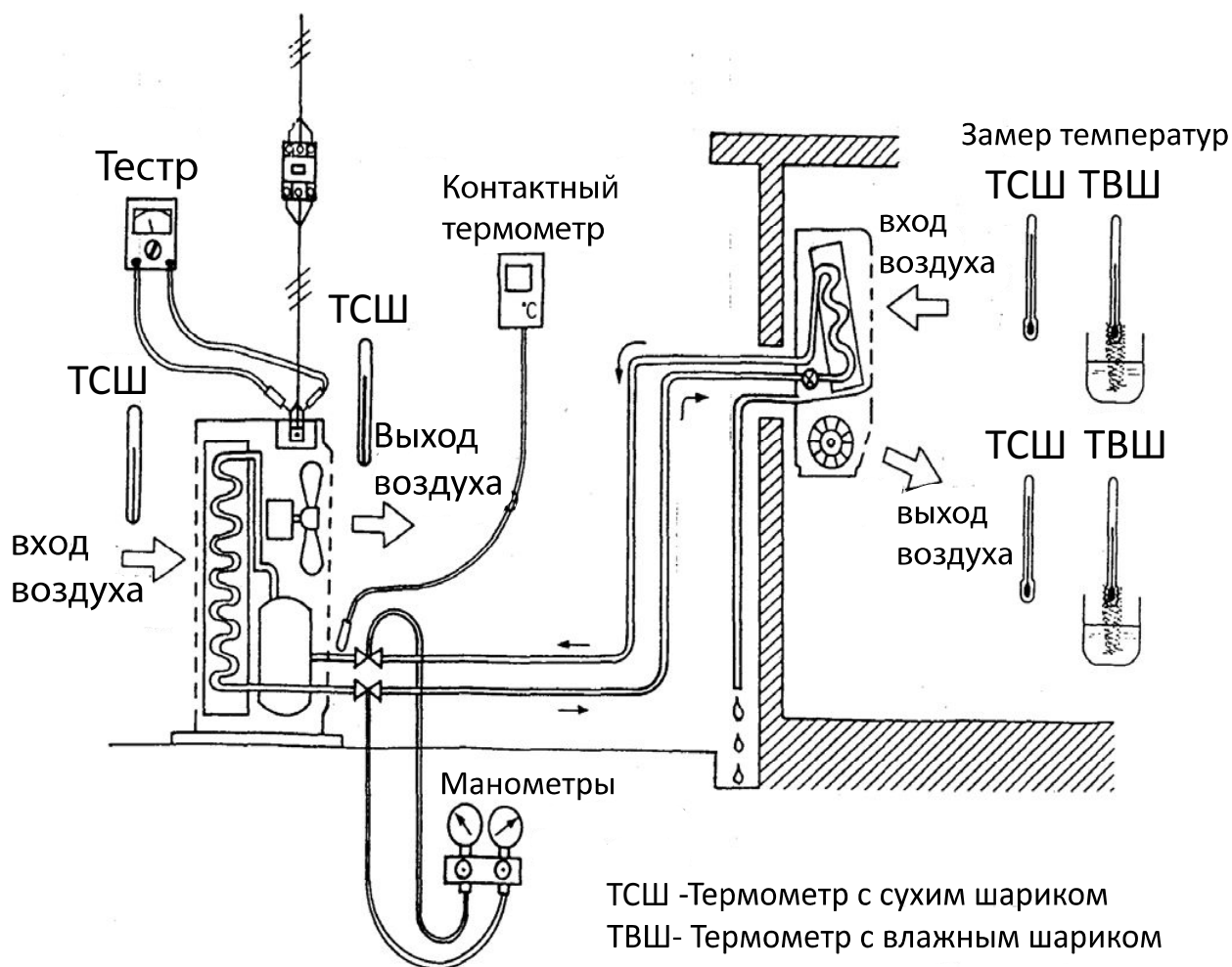
Рис. 8.1. Измеряемые параметры и применяемые приборы
