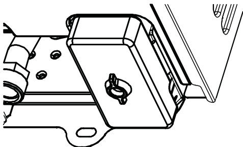
Рис. 6 Батарейный блок
