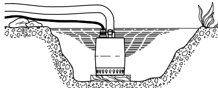
Նկար 6 Սալի վրա տեղադրված պոմպ
