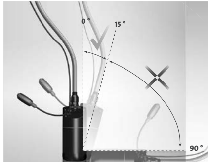
8-сүр. SB, SBA соркысмаcылар/орнотмолордун абалы
