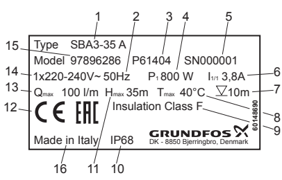
Նկար 1 Ֆիրմային վահանակի օրինակ
