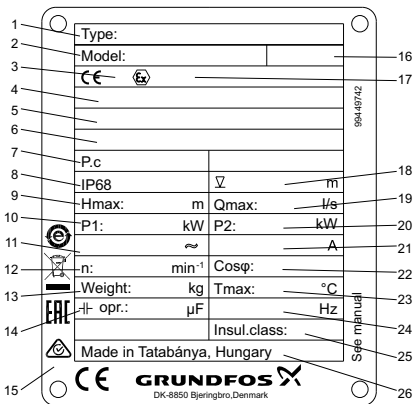
Рис. 1 Фирменная табличка
