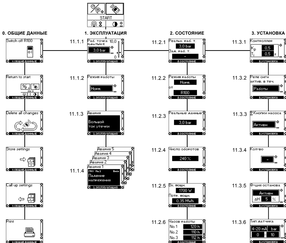
Рис. 26 Обзор меню
