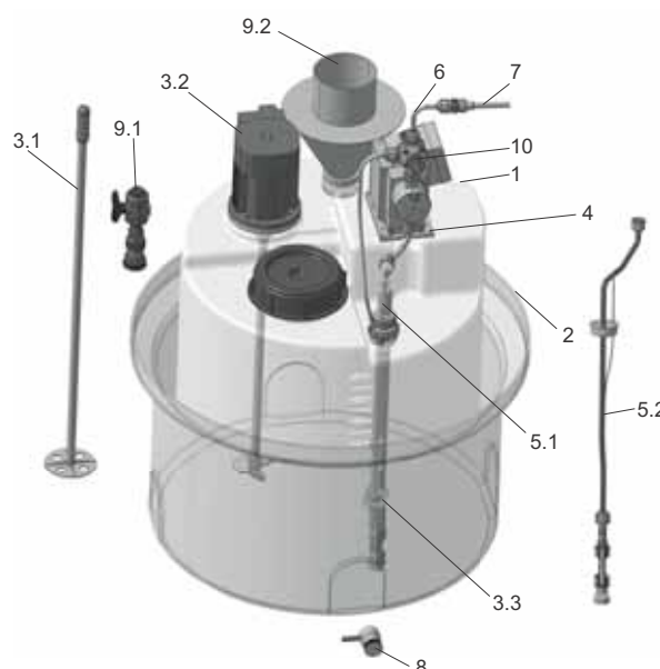
Рис. 7 Станция (пример)
