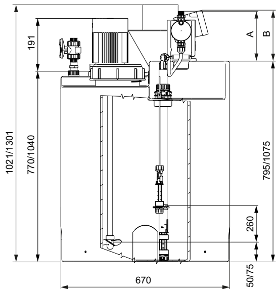
Рис. 3 Станция 200 / 300 л
