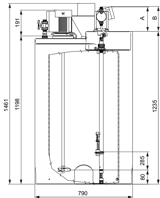
Рис. 4 Станция 500 л
