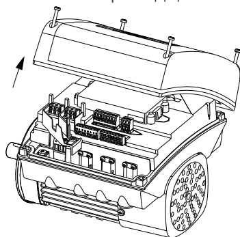
13-сур. Клеммалы қораптың қақпағының шешілуі
