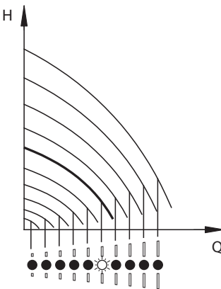
Рис. 31 Насос в режиме управления с постоянной характеристикой
