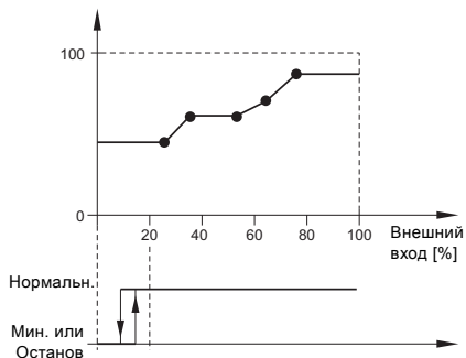
Рис. 62 Таблица влияни. с остан. у мин.
