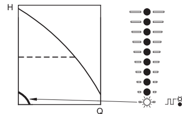
Рис. 33 Эксплуатация при минимальной характеристике
