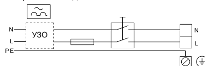
18-сур. Электрқорегінің ажыратқышы, ерігіш сақтандырғышы және қосымша қорғанышы бар электр қозғалтқышты желіге жалғаудың үлгісі
