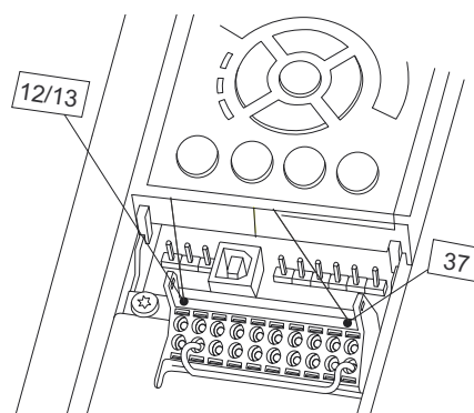
Рис. 12 Снятие перемычки
