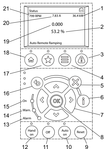
Рис. 24 Панель управления
