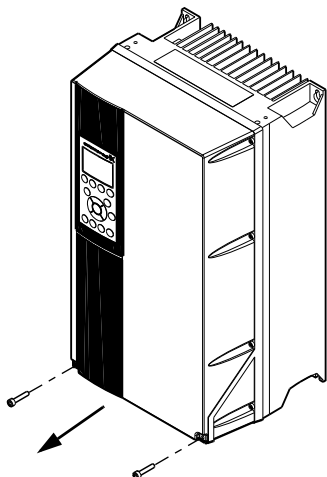
Рис. 14 Доступ к сигнальным релейным выходам, В2, С1
