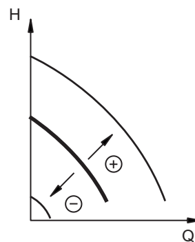
15-сур. Тұрақты сипаттамалы басқару режиміндегі сорғы
