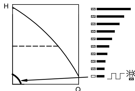
Рис. 14 Мин. характеристика
