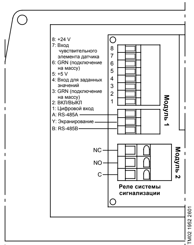
Рис. 4 Схема соединений
