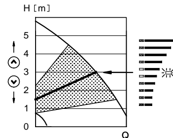
Рис. 11 Насос с пропорционально регулируемым давлением
