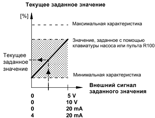
Рис. 19 Зависимость между фактическим значением и внешним сигналом заданного значения при режиме эксплуатации с постоянной характеристикой
