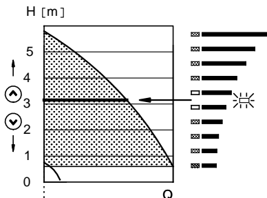
Рис. 17 Насос с регулированием постоянного давления
