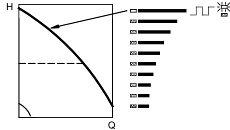
Рис. 18 Макс. характеристика
