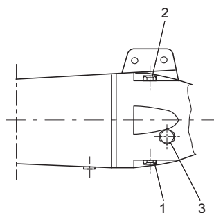
Рис. 15 Редуктор
