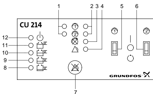
Рис. 4 Панель управления модуля CU 214
