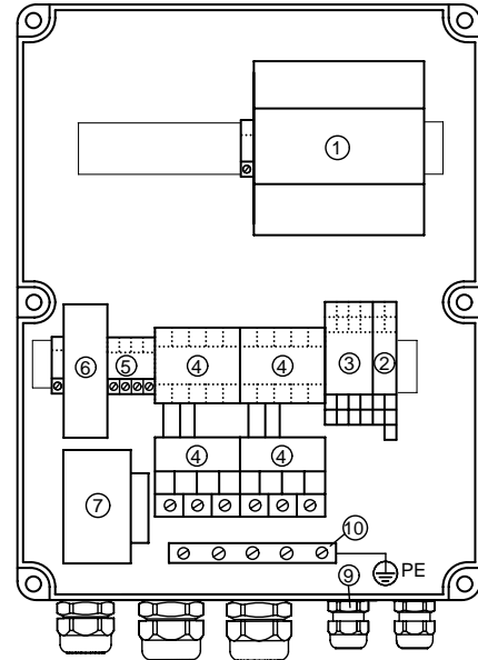
Рис. 11 Внутренняя компоновка шкафа LCD 110
