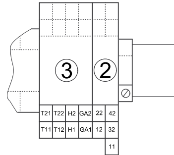
Рис. 12 Расположение клемм поз. 2 и 3
