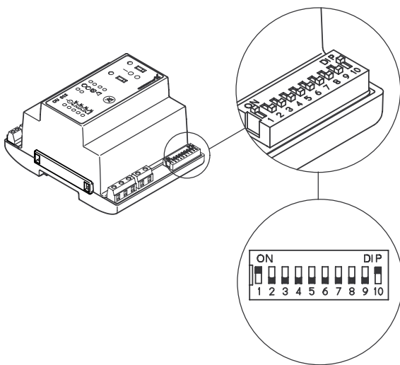
Рис. 6 Модуль CU 214 с микропереключателем
