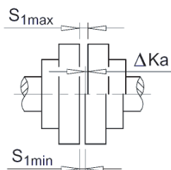
Черт. 23: смещение муфты
