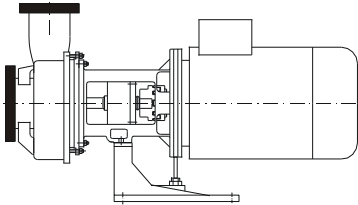
Черт. 13: MAXA Adapta® на чугунной опоре
