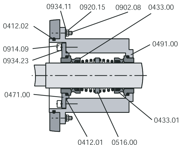
Черт. 11: двойное контактное уплотнение «Tandem», посадка L1K
