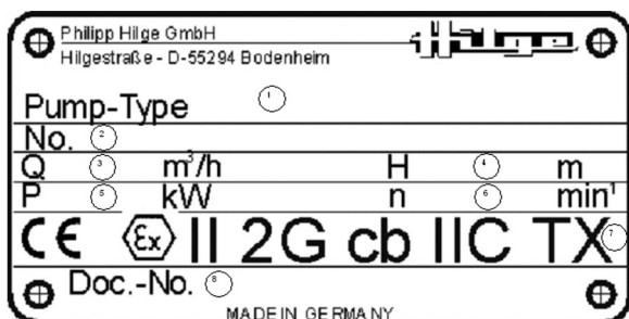
Черт. 1: образец фирменной таблички
